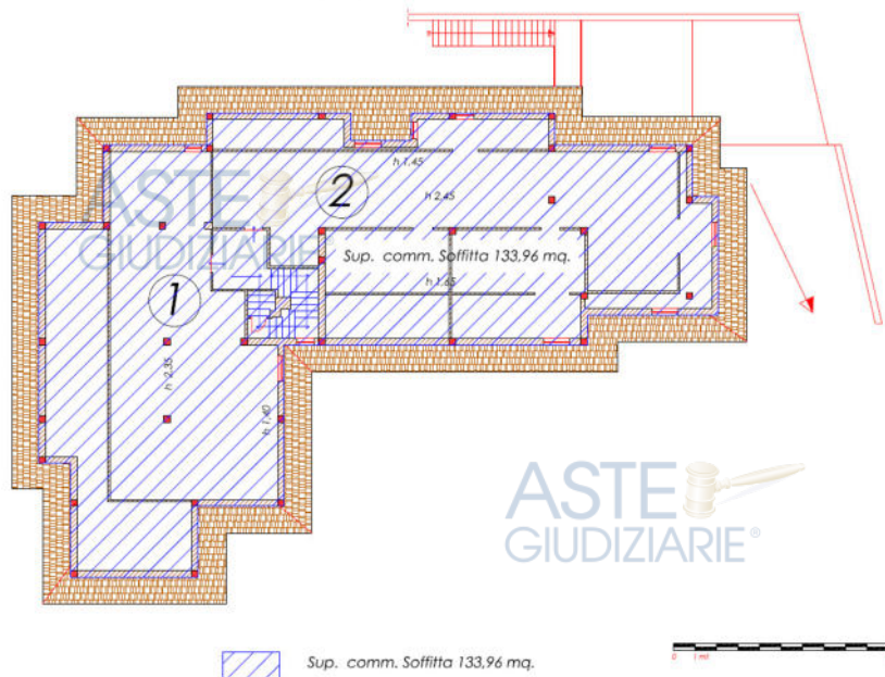
Pianta soffitta
