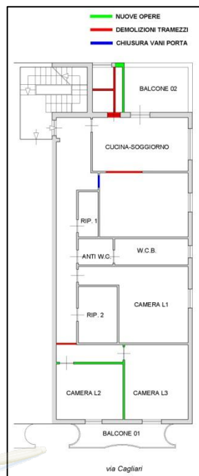
Pianta stato di fatto con indicazione delle difformità - All. 6
