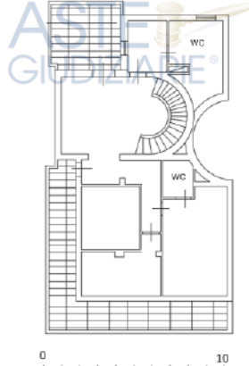
Rilievo dello stato dei luoghi piano terra e piano primo (All. 6)
