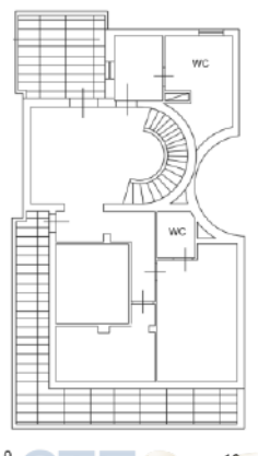
Ricostruzione planimetria catastale piano terra e piano primo (All. 9)
