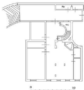
Planimetria dello stato futuro piano secondo ed S1 (All. 9)
