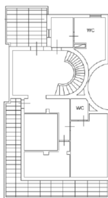
Planimetria di rilievo attuale piano secondo ed S1 (All. 6)
