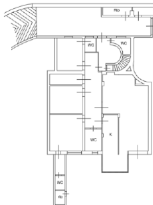
Planimetria di rilievo attuale piano secondo ed S1 (All. 6)
