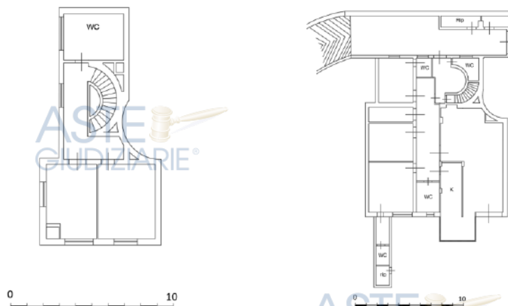
Rilievo dello stato dei luoghi piano secondo ed S1 (All. 6)
