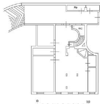
Ricostruzione planimetria catastale piano secondo ed S1 (All. 9)
