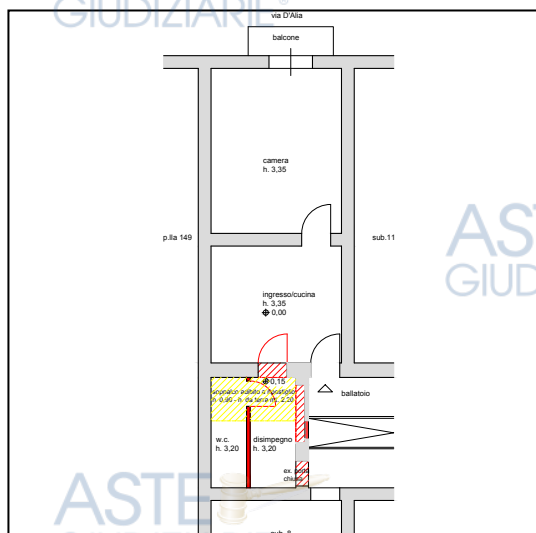
Planimetria di rilievo attuale dei luoghi con l'indicazione grafica delle difformità edilizio- urbanistiche rispetto alla planimetria catastale d'impianto (All.15)
