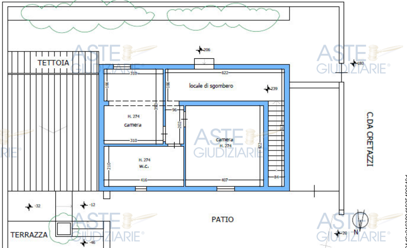
Rilievo dello stato di fatto – piano terra
