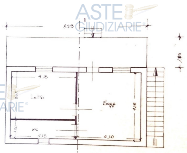
Planimetria allegata al Condono (47/85)
