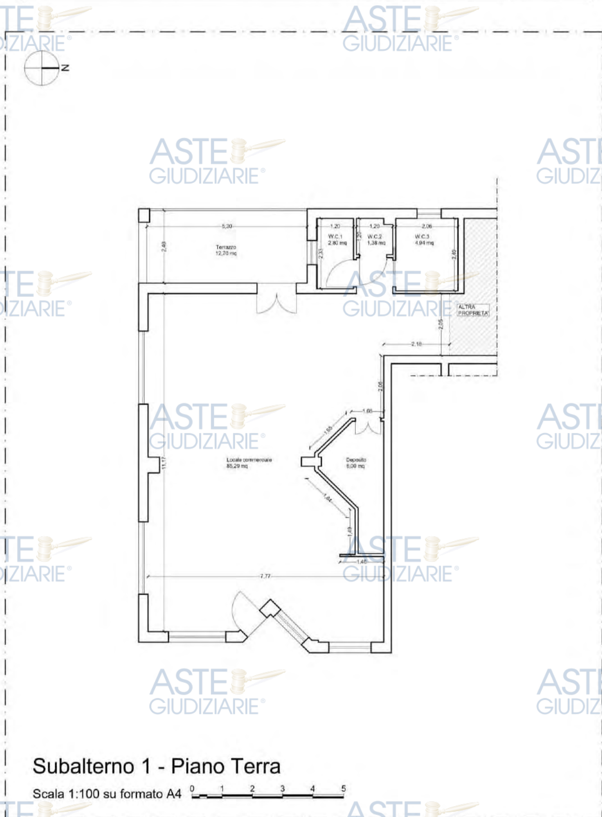
Figura 4 – Planimetria dello stato di fatto – Subalterno 1 – Piano Terra
