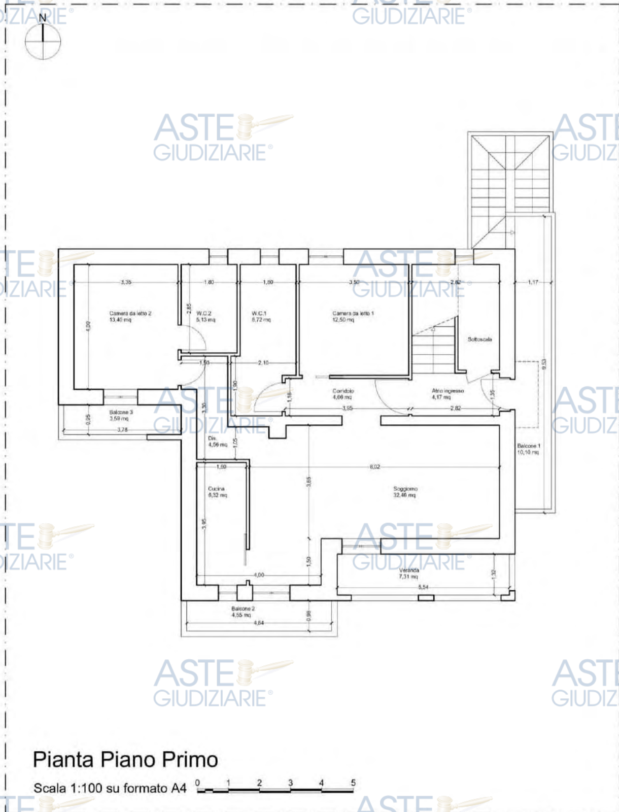
Figura 8 – Planimetria dello stato di fatto – Pianta Piano Primo
