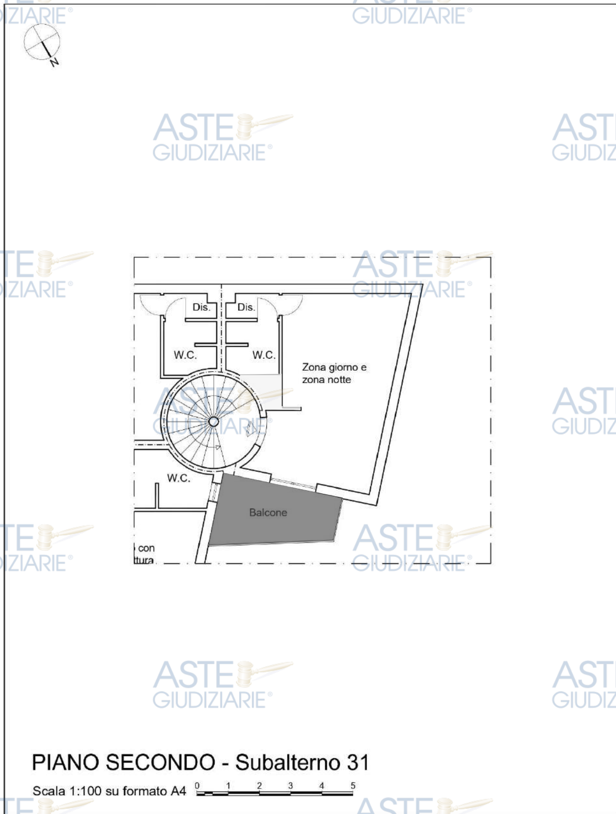
Figura 84 – Planimetria dello stato di fatto – Subalterno 31 – Piano Secondo
