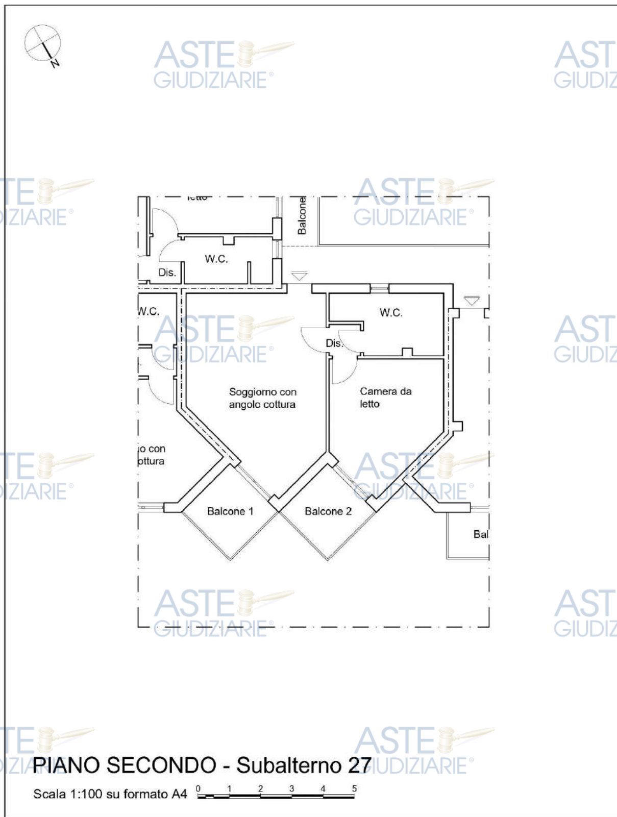
Figura 80 – Planimetria dello stato di fatto – Subalterno 27 – Piano Secondo
