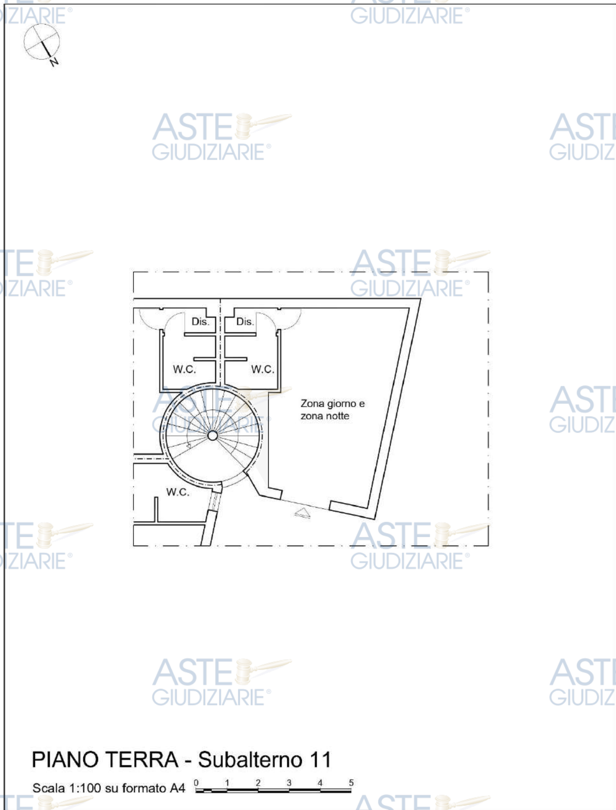
Figura 58 – Planimetria dello stato di fatto – Subalterno 11 – Piano Terra
