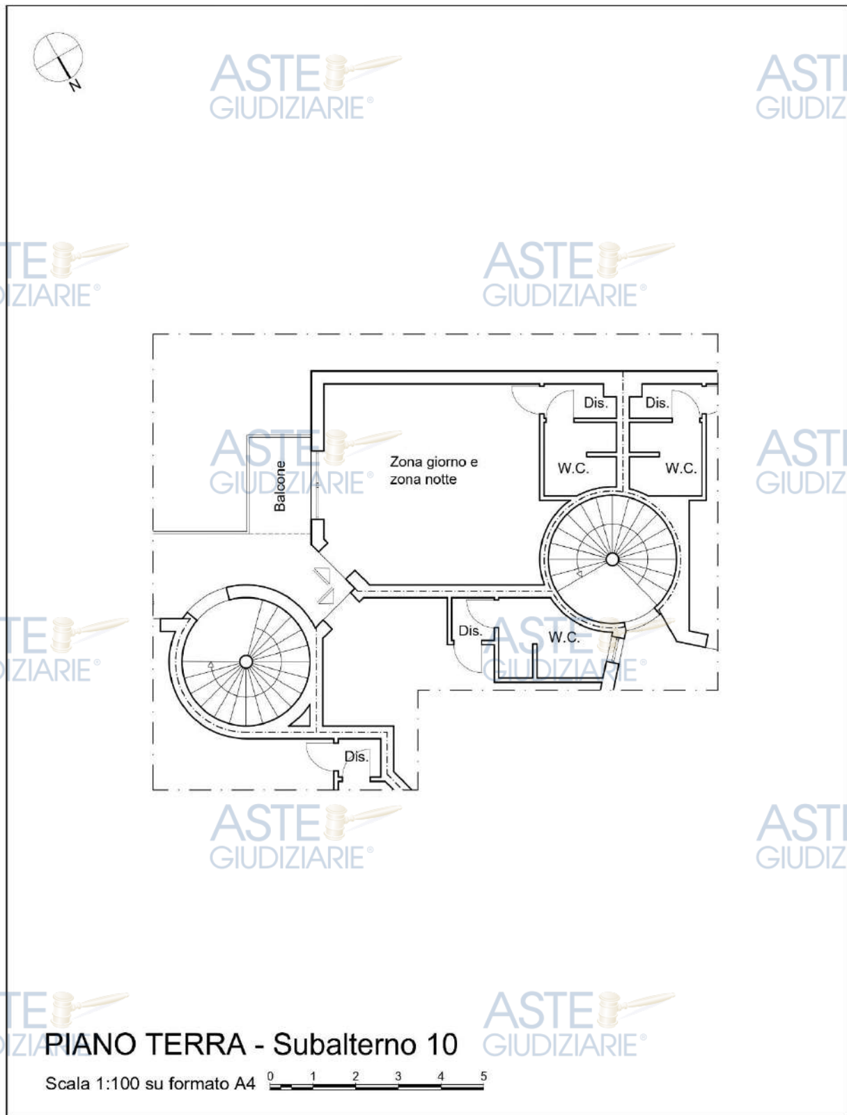
Figura 56 – Planimetria dello stato di fatto – Subalterno 10 – Piano Terra
