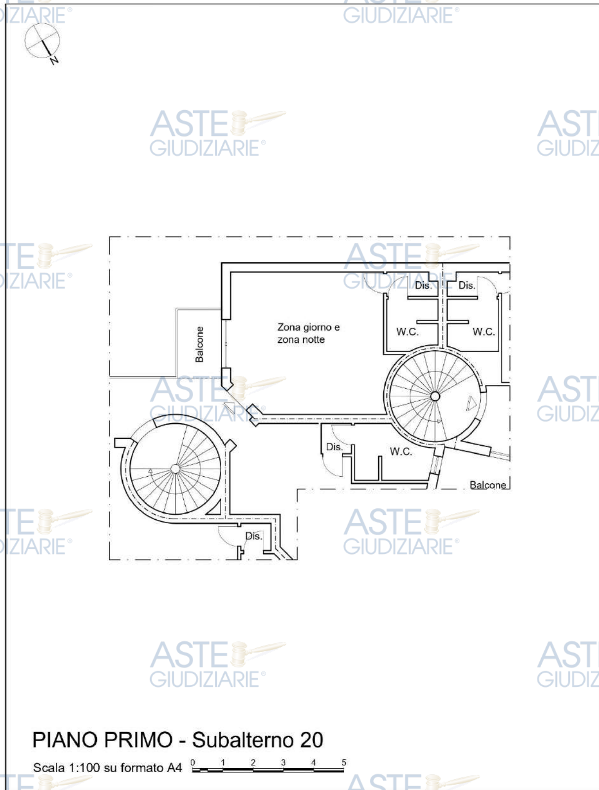
Figura 24 – Planimetria dello stato di fatto – Subalterno 20 – Piano Primo
