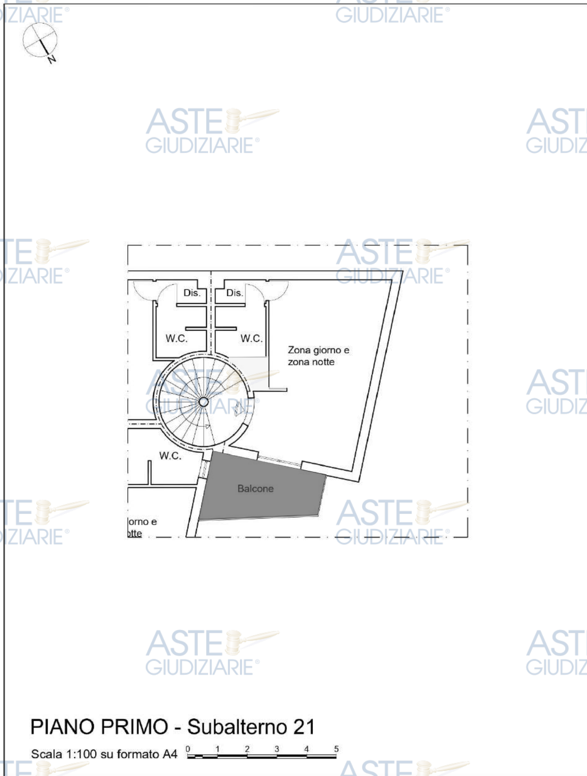
Figura 73 – Planimetria dello stato di fatto – Subalterno 21 – Piano Primo
