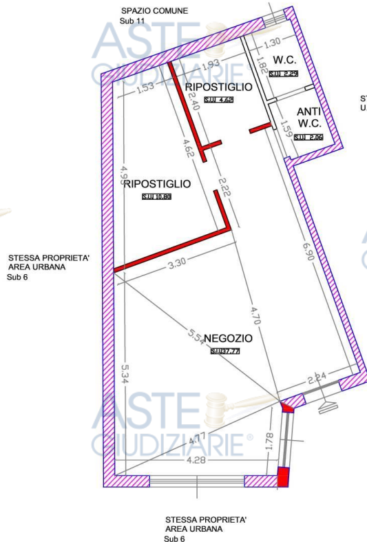
FOTO 5 - Pianta del locale commerciale dopo rilievo primo accesso
