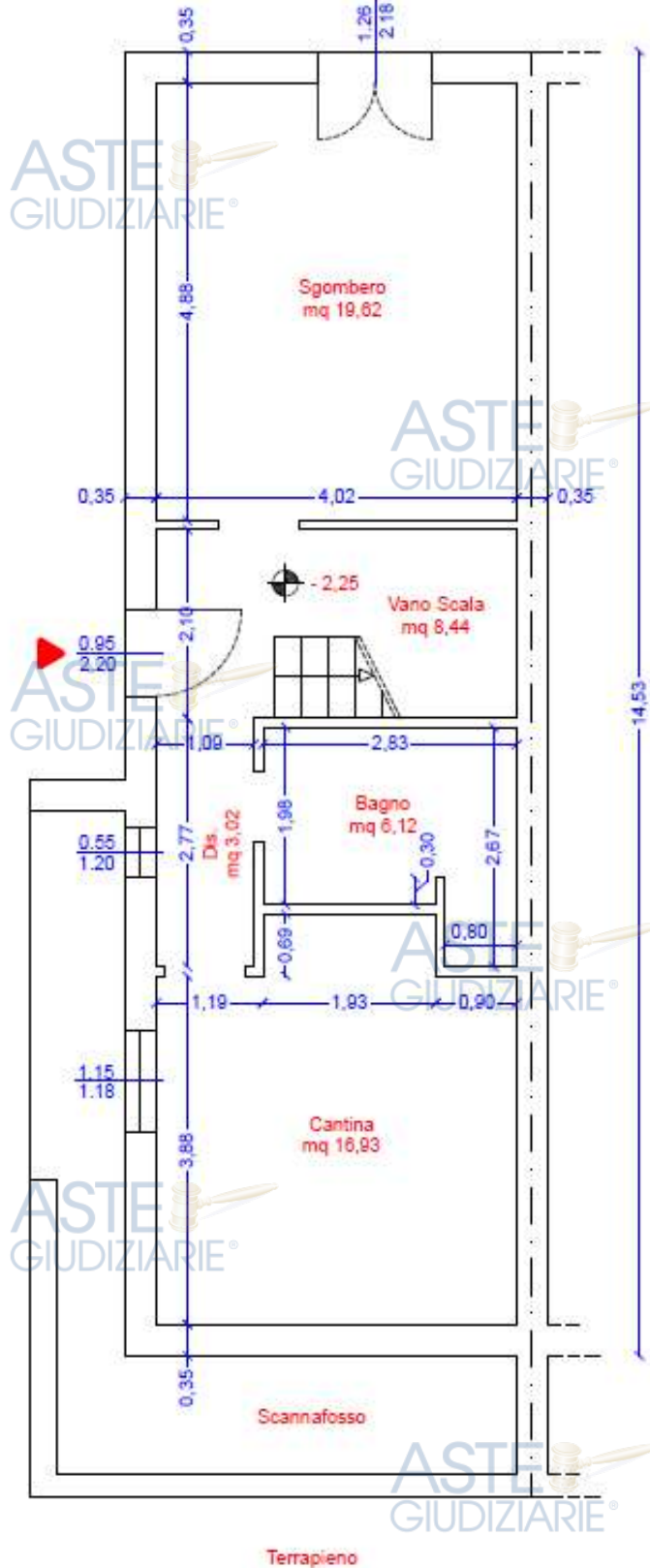
Figura 15 - Rilievo sub. 1 piano seminterrato, fuori scala. H mt 2,50
