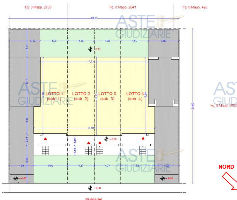
Figura 14 - Rilievo del lotto e confini. Fuori scala
