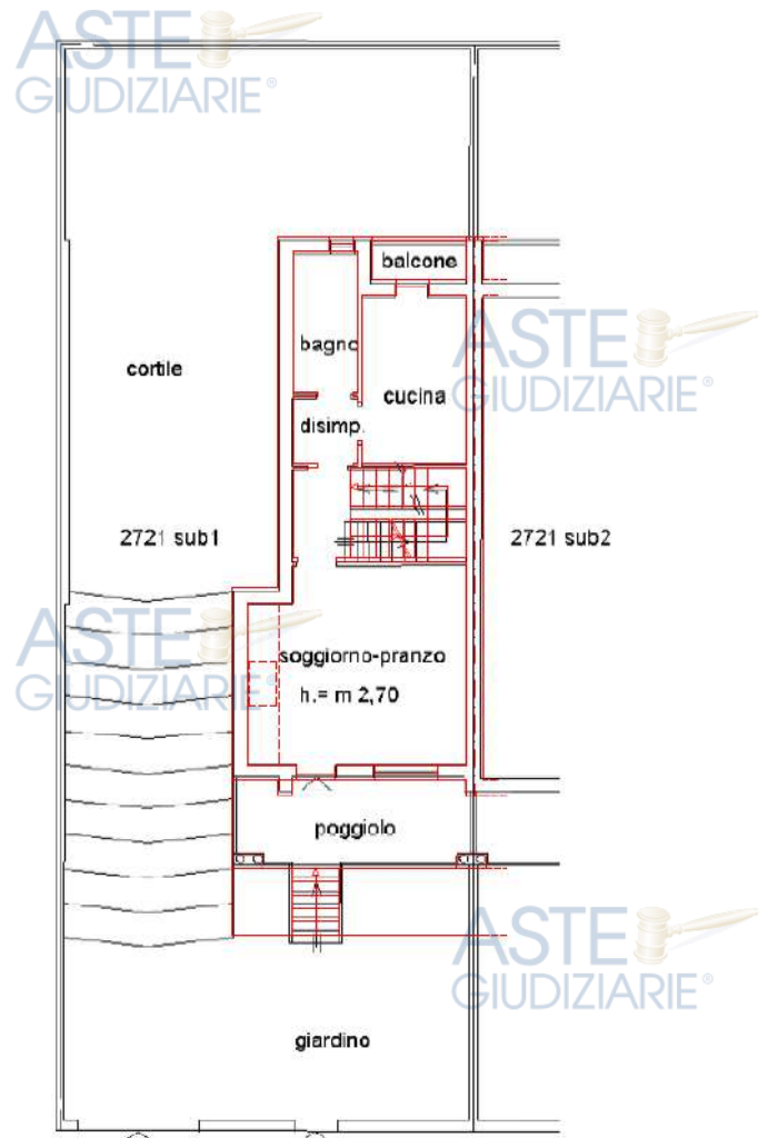
Figura 67 – Sovrapposizione rilievo con planimetria catastale in atti (fuori scala). Piano terra
