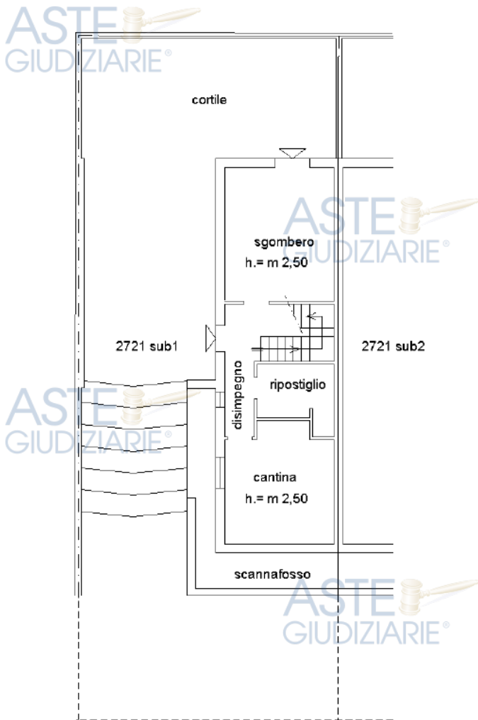
Figura 63 – Stralcio planimetria catastale in atti (fuori scala). Piano seminterrato
