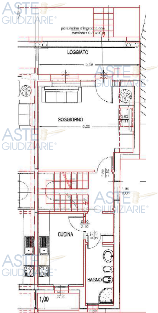
Figura 70 - Sovrapposizione progetto-rilievo. Piano T, fuori scala
