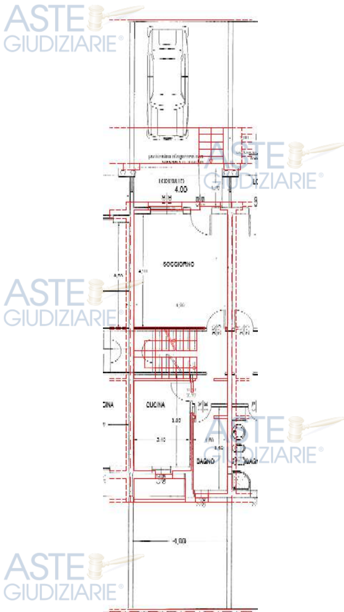
Figura 66 - Sovrapposizione progetto-rilievo. Piano T, fuori scala
