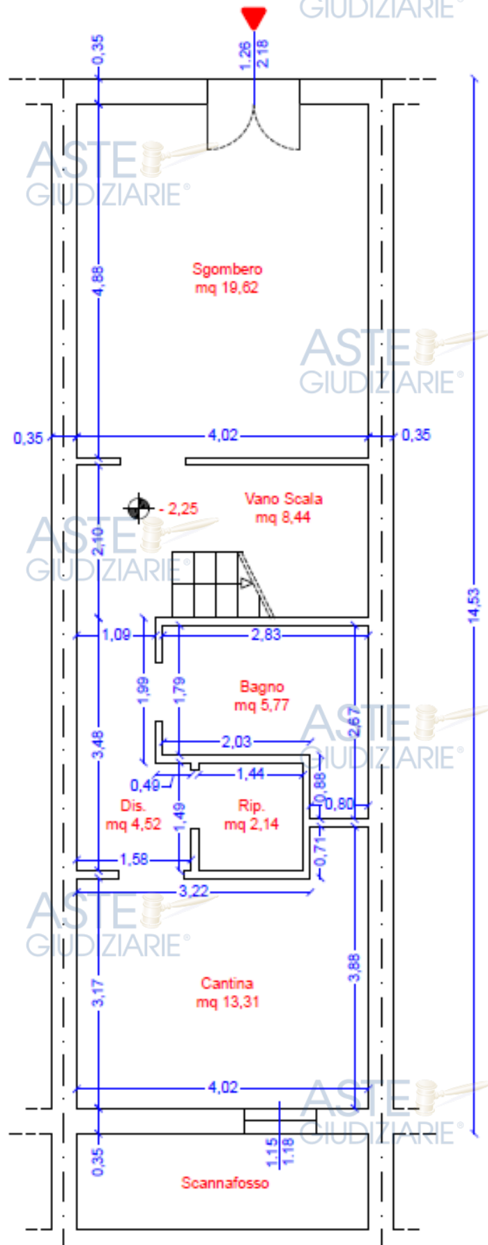
Figura 15 - Rilievo sub. 3 piano seminterrato, fuori scala. H mt 2,50
