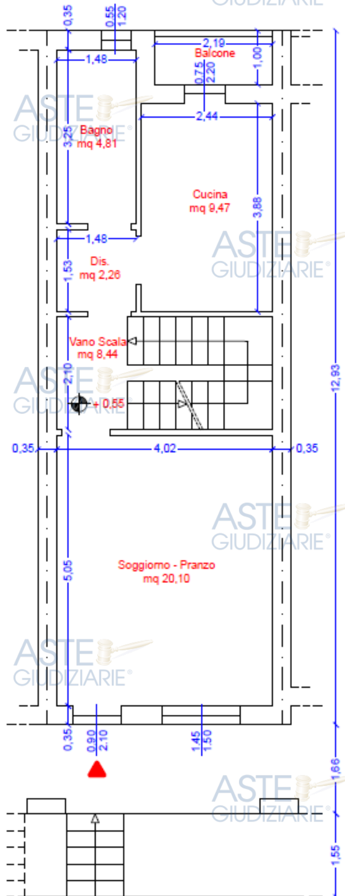
Figura 16 - Rilievo sub. 3 piano terra, fuori scala. H mt 2,70
