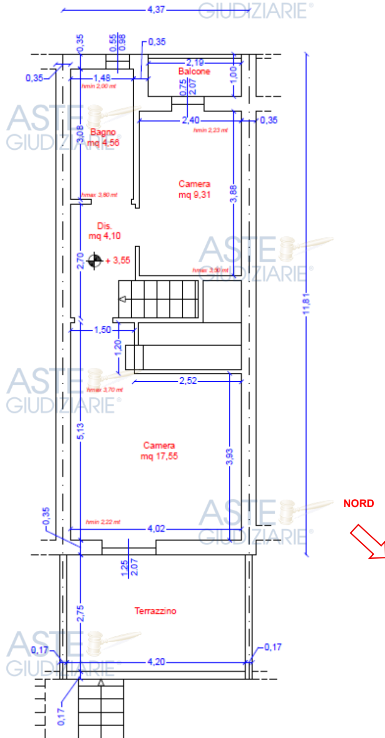
Figura 17 - Rilievo sub. 3 piano primo, fuori scala. H varie
