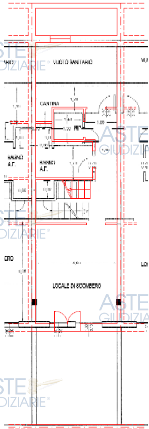
Figura 65 - Sovrapposizione progetto-rilievo. Piano S1, fuori scala
