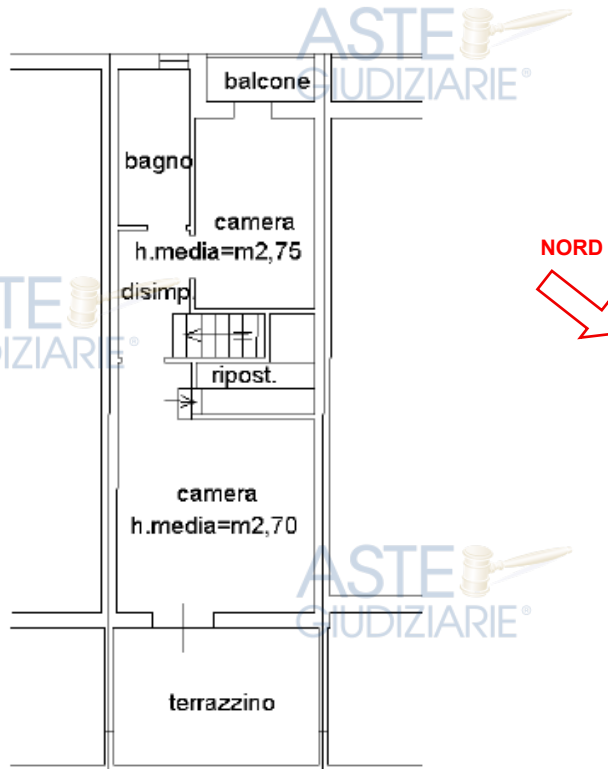
Figura 61 – Stralcio planimetria catastale in atti (fuori scala). Piano primo
