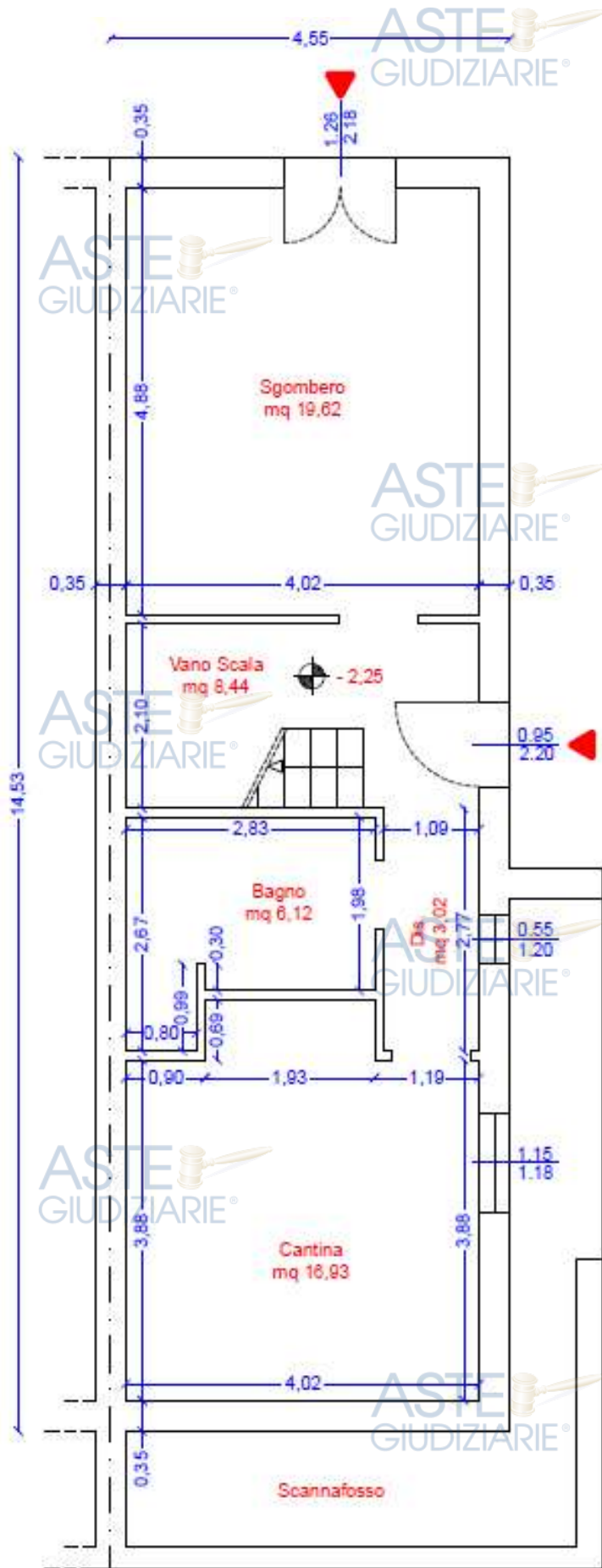
Figura 15 - Rilievo sub. 4 piano seminterrato, fuori scala. H mt 2,50
