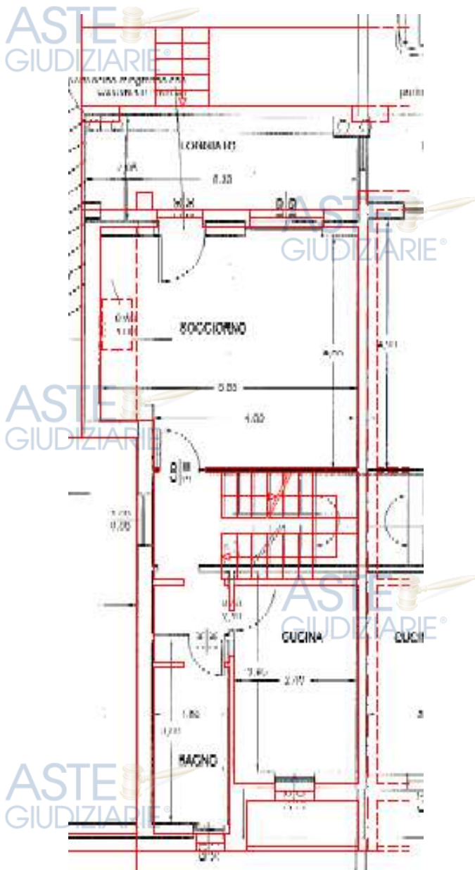
Figura 68 - Sovrapposizione progetto-rilievo. Piano T, fuori scala
