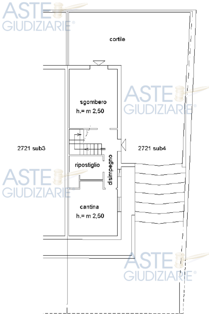
Figura 61 – Stralcio planimetria catastale in atti (fuori scala). Piano seminterrato
