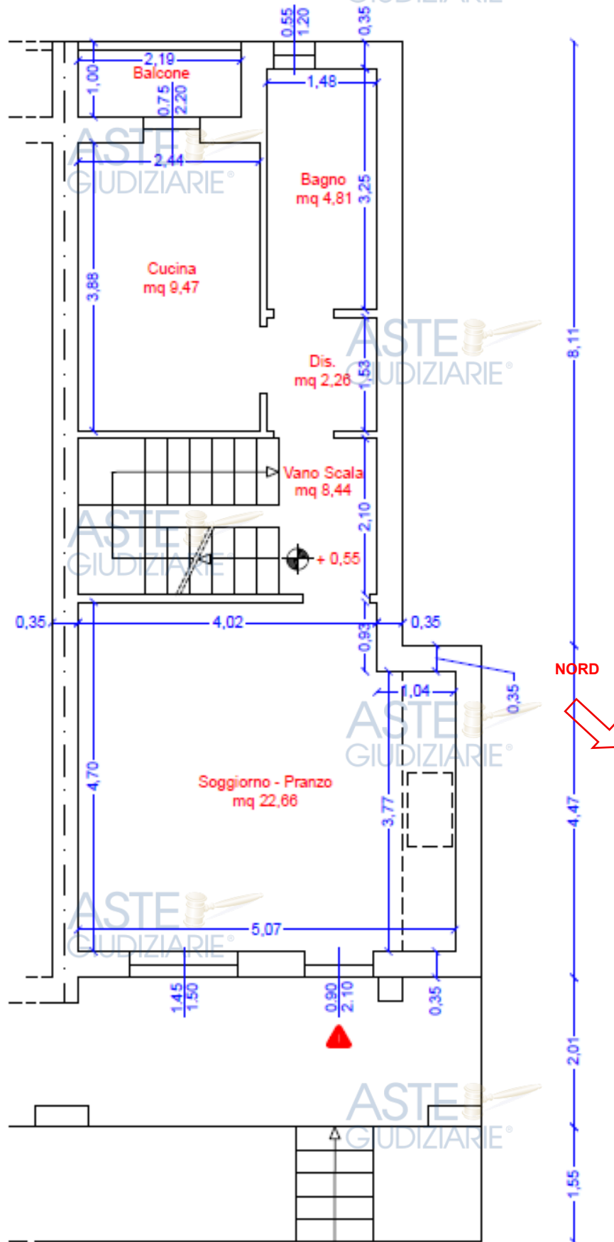
Figura 16 - Rilievo sub. 4 piano terra, fuori scala. H mt 2,70
