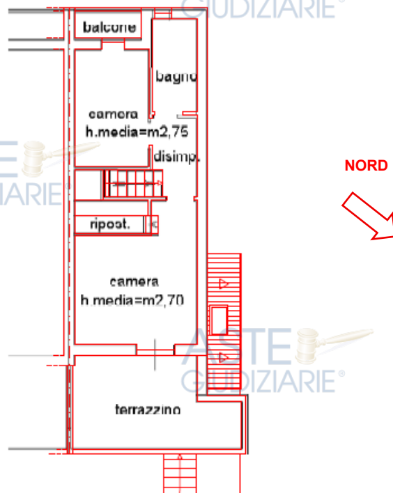
Figura 66 – Sovrapposizione rilievo con planimetria catastale in atti (fuori scala). Piano primo
