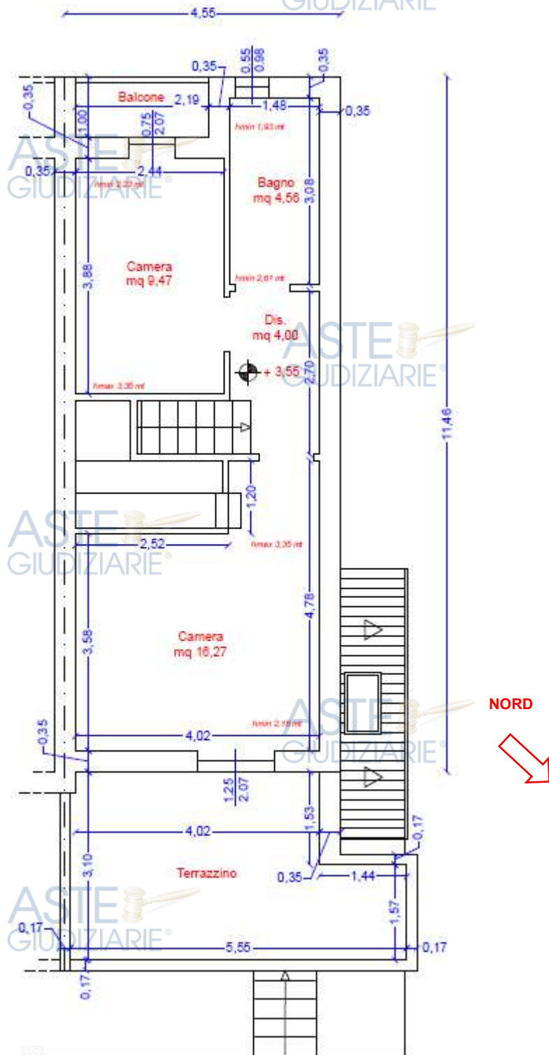
Figura 17 - Rilievo sub. 4 piano primo, fuori scala. H varie
