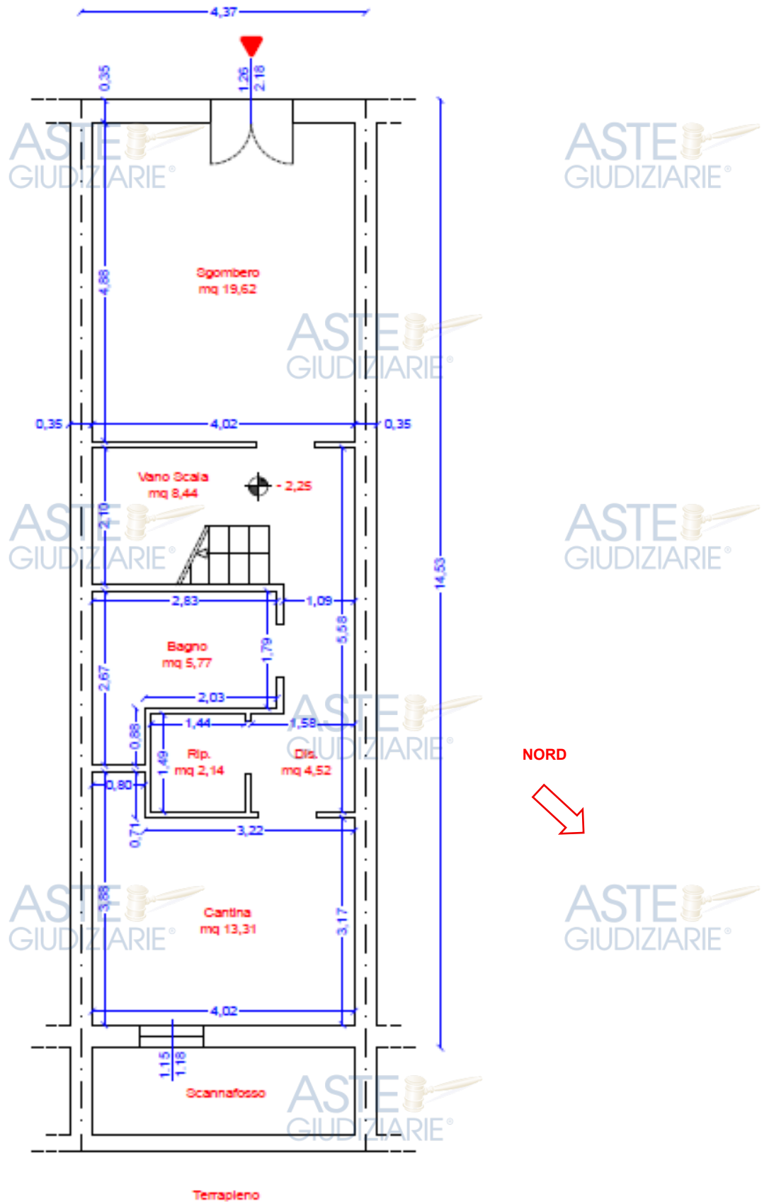
Figura 15 - Rilievo sub. 2 piano seminterrato, fuori scala. H mt 2,50
