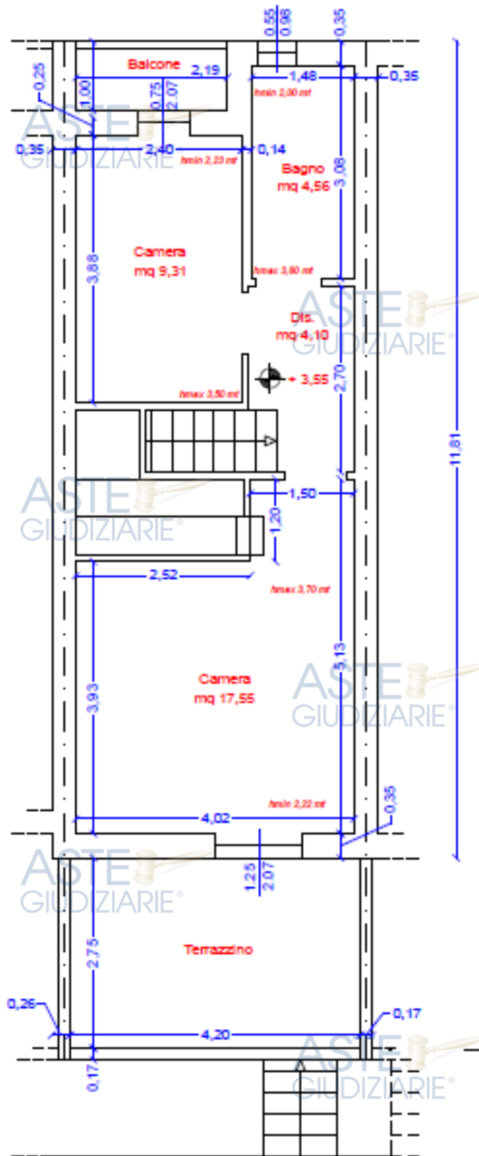
Figura 17 - Rilievo sub. 2 piano primo, fuori scala. H varie
