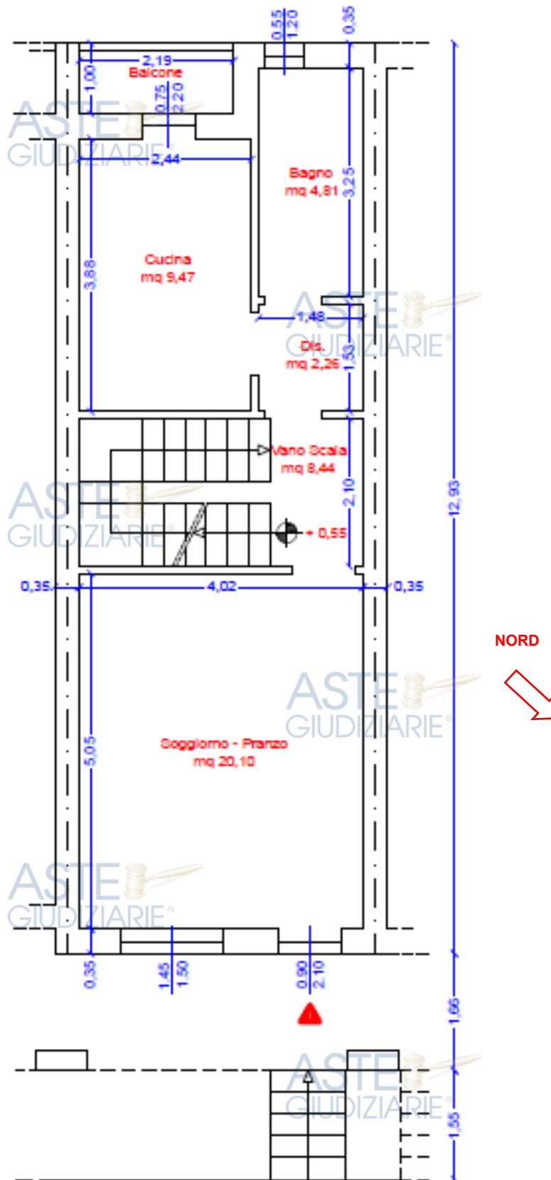
Figura 16 - Rilievo sub. 2 piano terra, fuori scala. H mt 2,70
