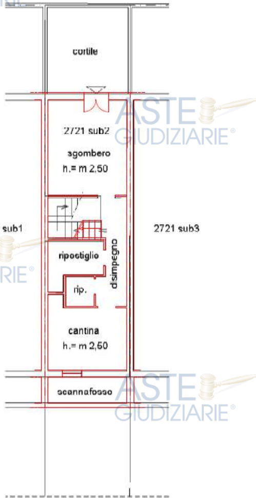
Figura 64 – Sovrapposizione rilievo con planimetria catastale in atti (fuori scala). Piano seminterrato
