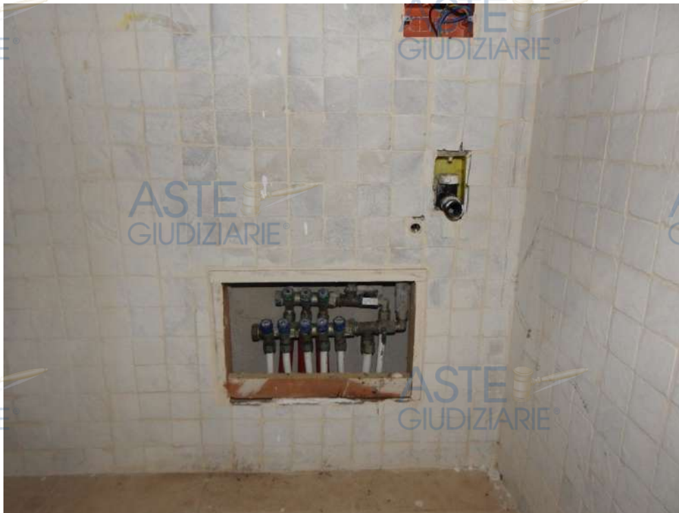
Figura 54 – Collettore impianto idrico piano seminterrato
