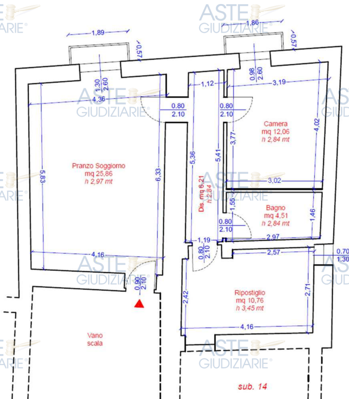
Figura 50 - Rilievo dello stato di fatto (fuori scala)
