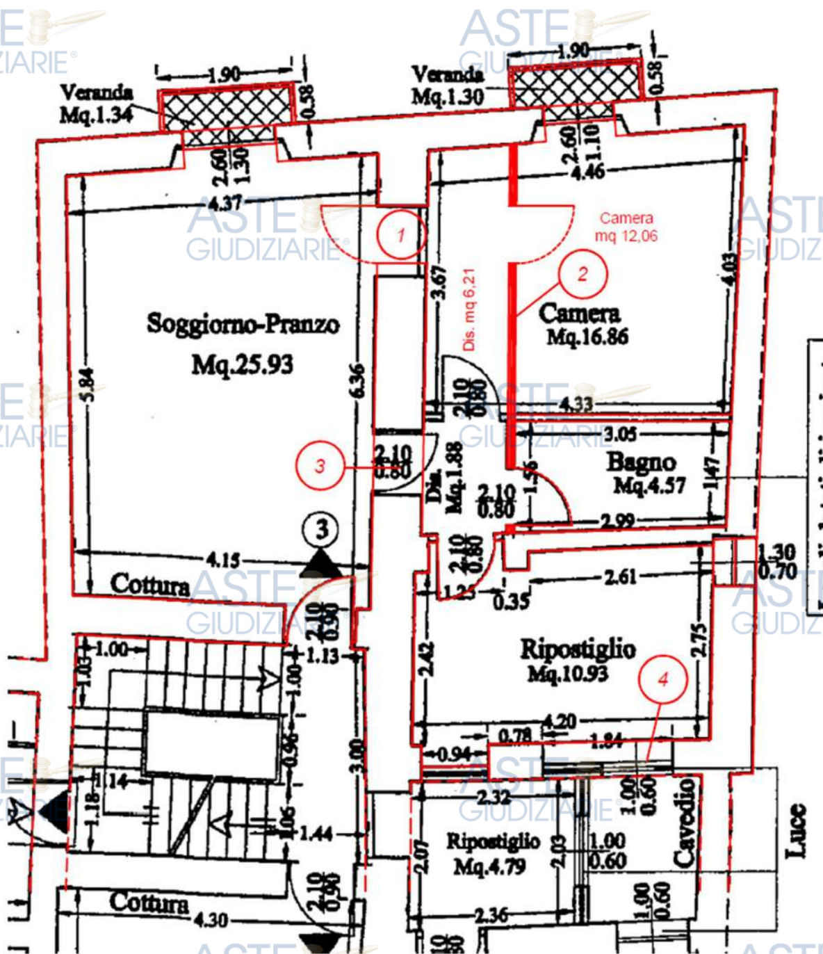
Figura 51 - Sovrapposizione dello stato di fatto su quello legittimo (fuori scala)
