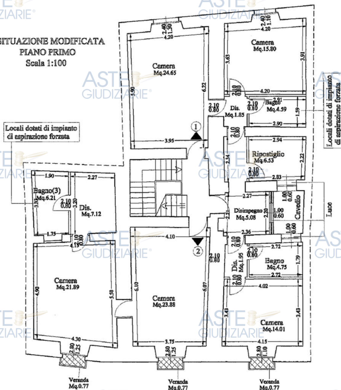
Figura 78 - Stralcio dell'ultimo progetto approvato. Aut. Ed. n. 105/2007 (fuori scala). Primo Piano
