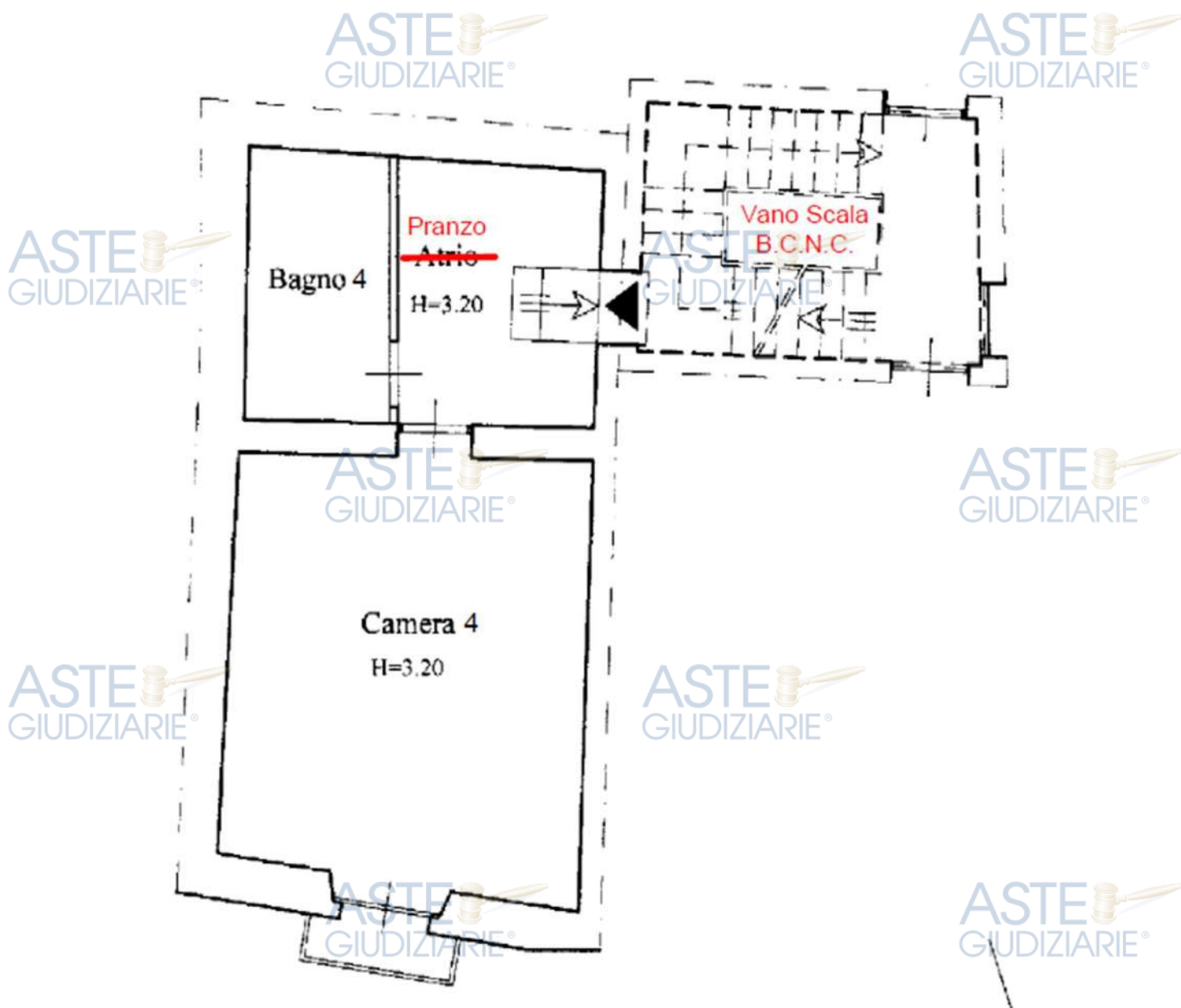
Figura 36 - Planimetria piano Secondo, fuori scala
