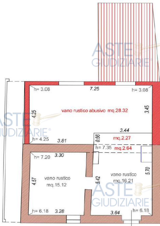
PIANTA PIANO 1°
