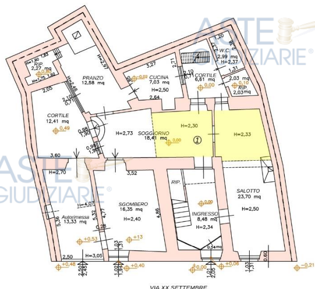
PIANTA PIANO TERRA SC. 1:100 RILIEVO ATTUALE
