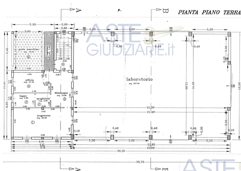
Planimetria del piano terra
