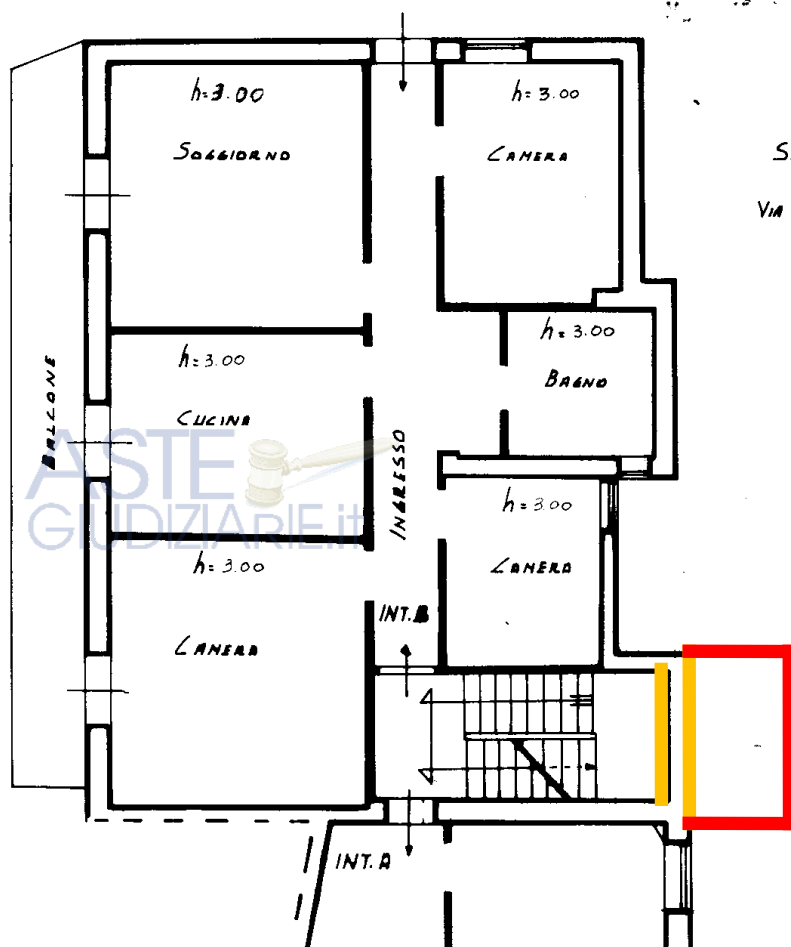
PIANTA 1° PIANO
