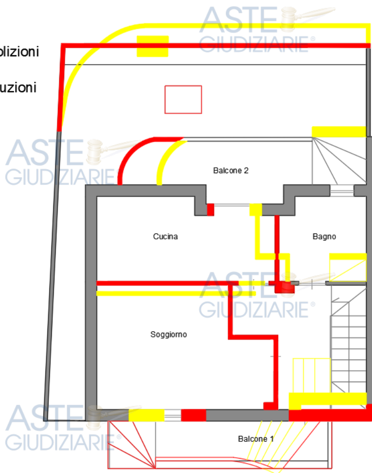
Figura 4 – Confronto Edilizio con Variante alla C.E. n. 40949/2005 – Pianta Piano Terra
