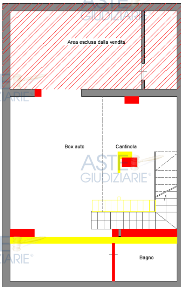
Figura 2 – Confronto catastale – Pianta piano seminterrato
