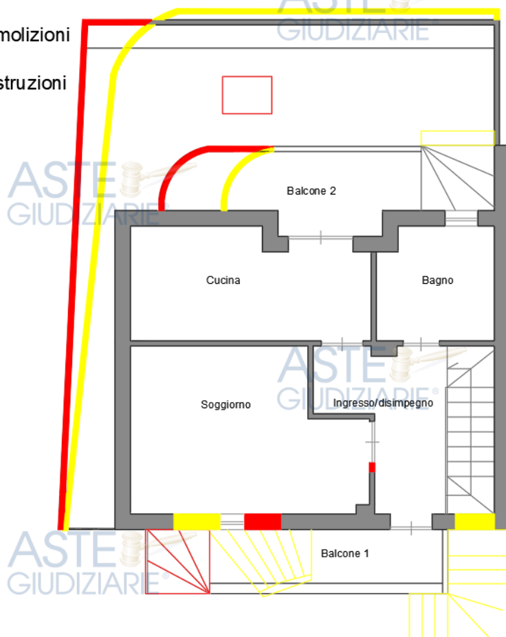
Figura 1 – Confronto catastale – pianta piano terra
