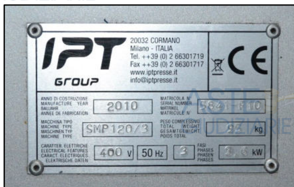
Foto 46: targhetta identificativa
