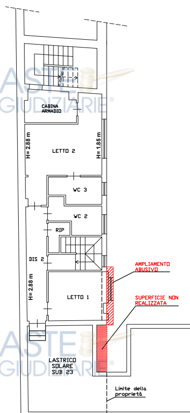
PLANIMETRIA APPARTAMENTO II PIANO DIFFORMITA' RILEVATE
