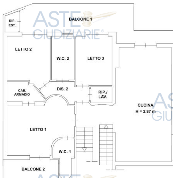
PLANIMETRIA APPARTAMENTO – PIANO SECONDO
