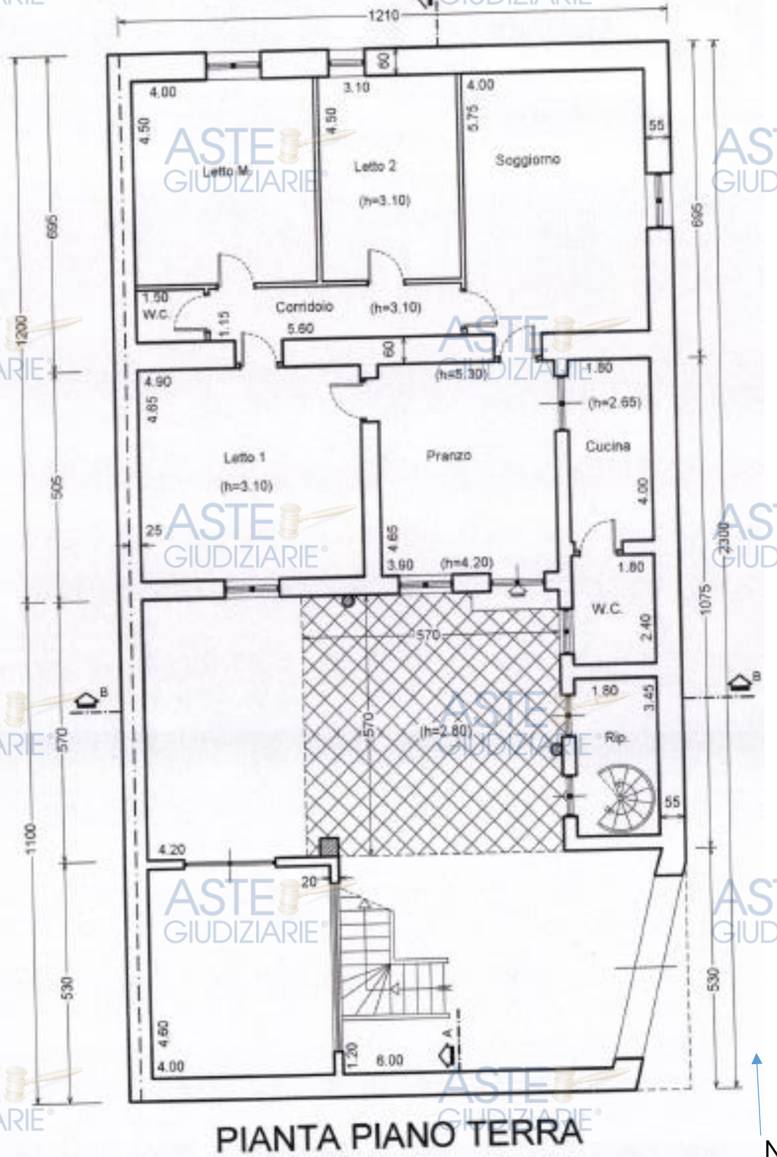
Planimetria principale
