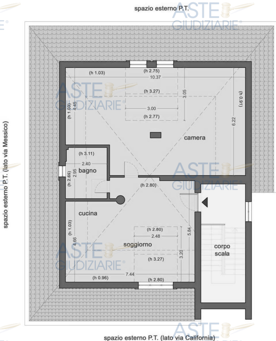
gr2.02: pianta stato di fatto PIANO TERZO (SOTTOTETTO)
