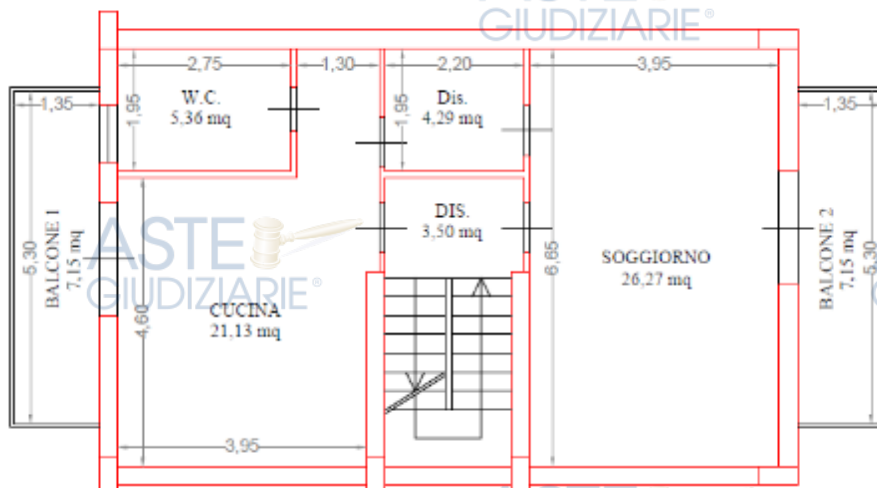
PIANTA PIANO PRIMO H=2,77m
