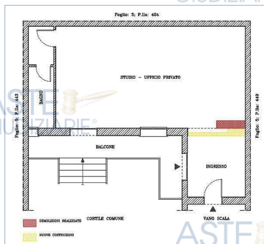
Stralcio della planimetria dello stato reale dei luoghi con indicazione grafica delle difformità catastali
