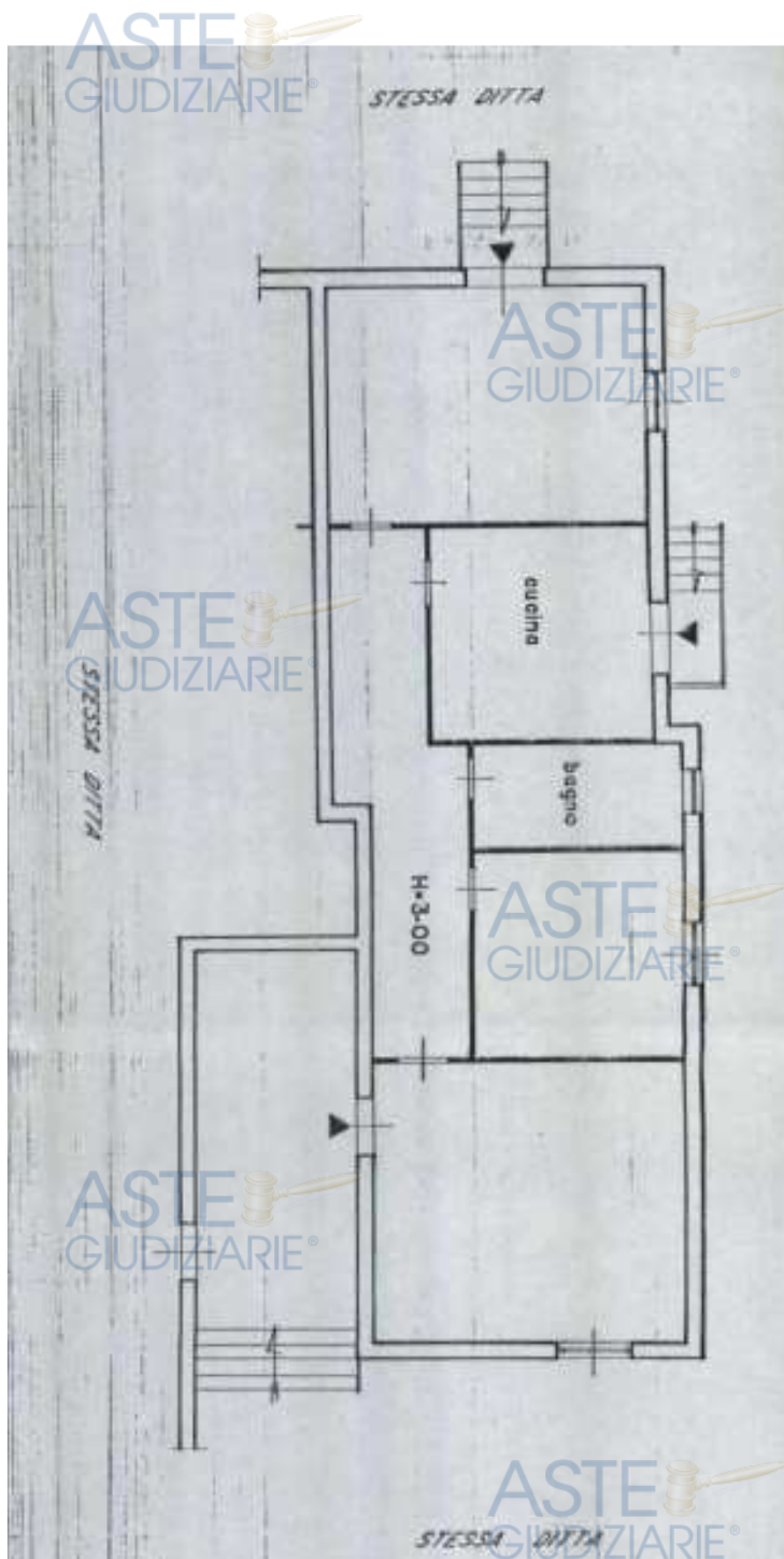
Fig. n° 3 – In questa planimetria non è presente il terrazzo dove in seguito è stata realizzata la cucina
