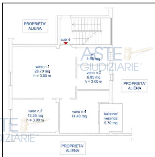
Plan. stato dei luoghi del 11/06/2025
