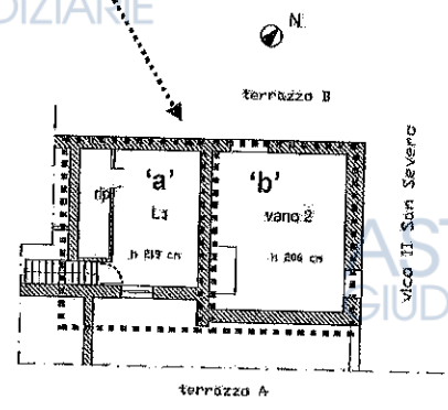
Planimetria dello stato di fatto
