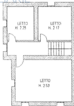
PIANO PRIMO
