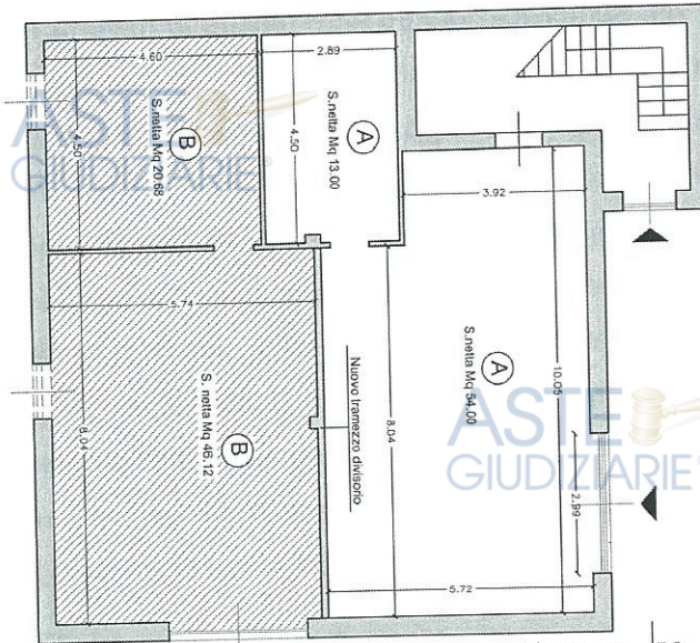
Pianta Piano Terra FG 29 PLLA 72 SUB 1
