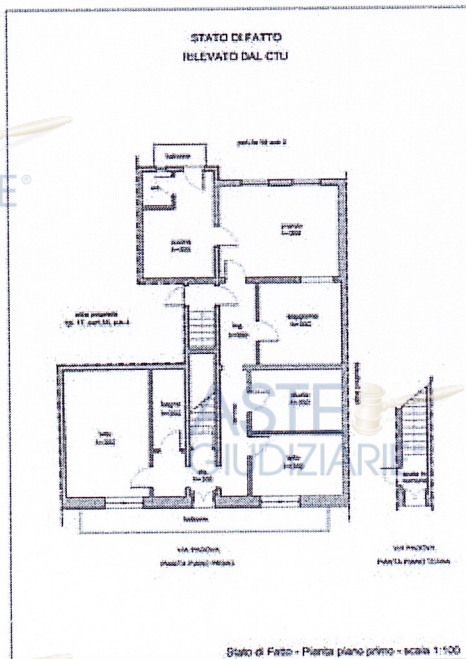
STATO DI FATTO P. PRIMO RILEVATO DAL CTU
