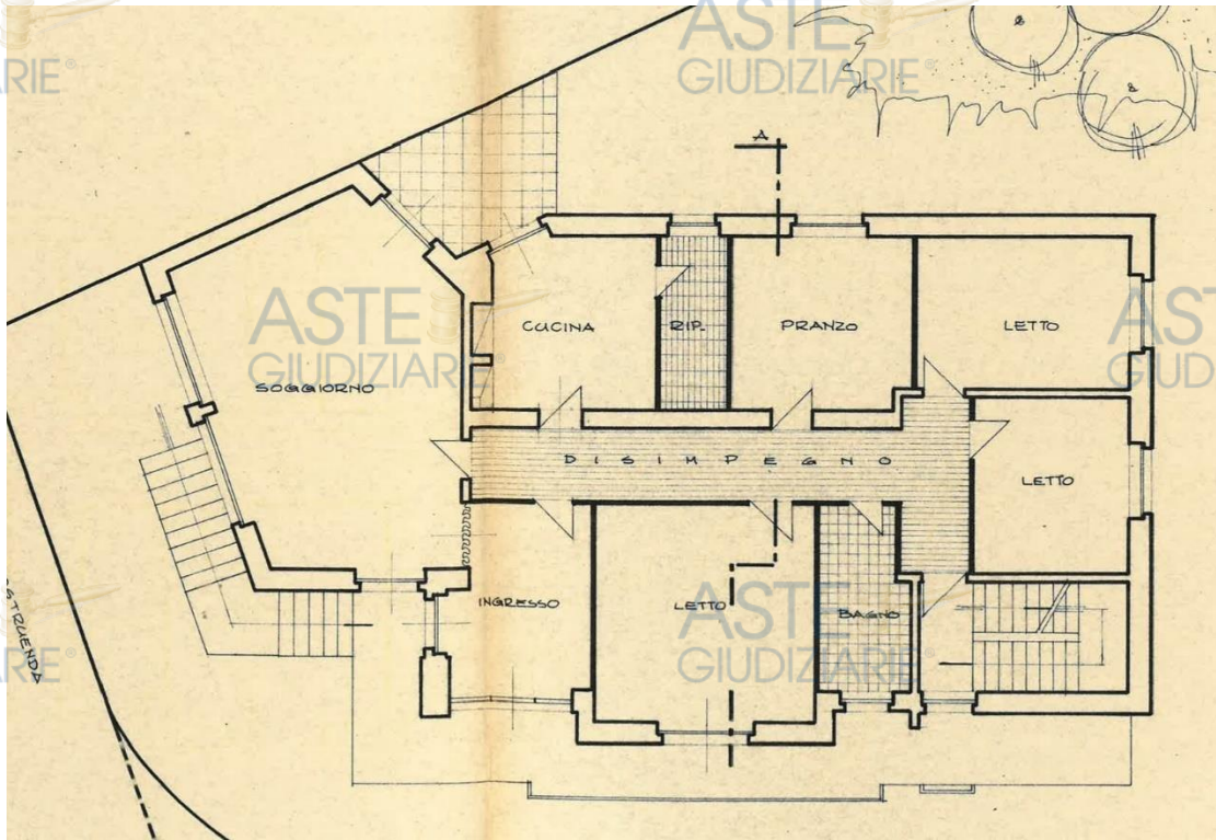
Elaborato legittimato dal titolo edilizo. Pianta primo piano
