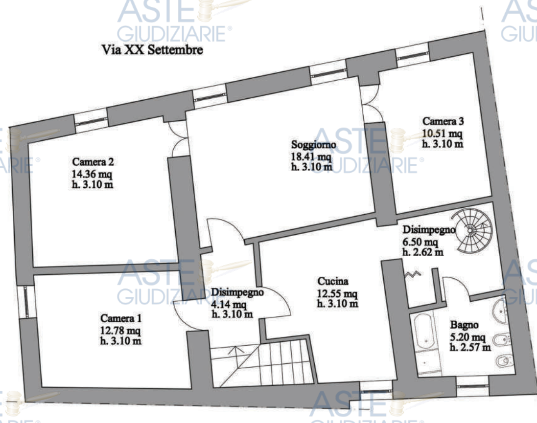
PIANO PRIMO
