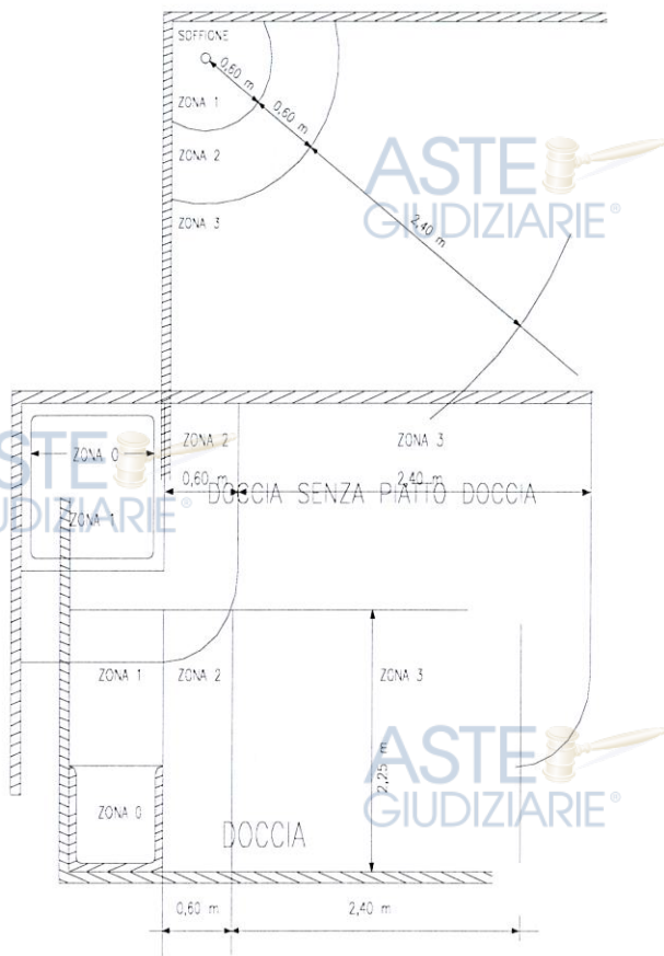
VASCA DA BAGNO
