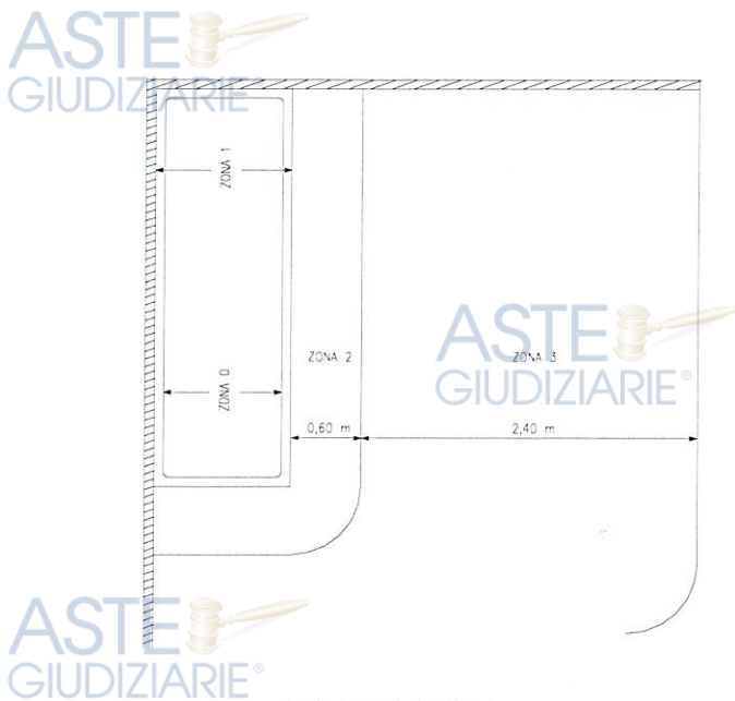
VASCA DA BAGNO
