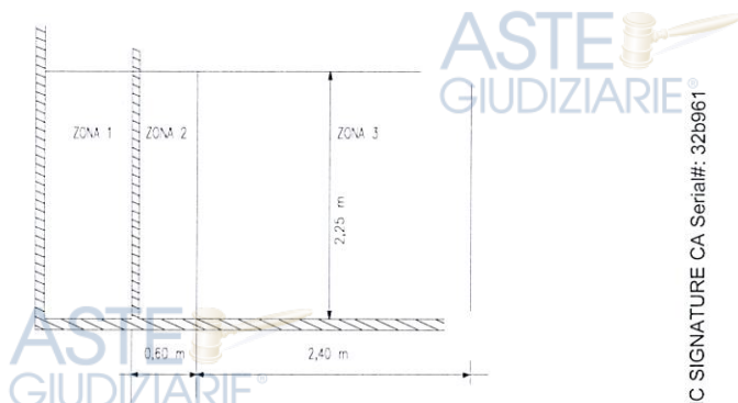
DOCCIA SENZA PIATTO, MA CON PARETE FISSA
