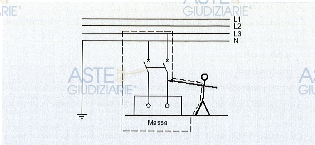
Esempio di contatto di diretto
