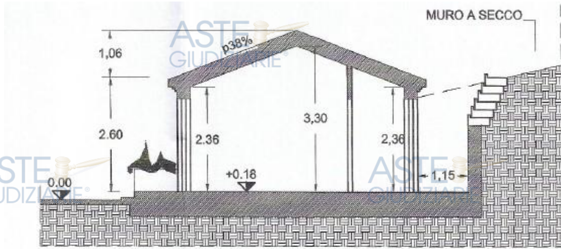
Sezione B-B'
