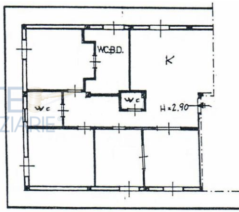
Pianta unità immobiliare come stato di fatto (da sopralluogo del 12/11/2012)
