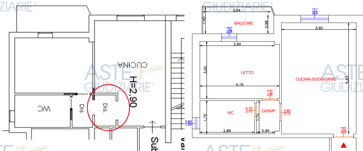
Figura 70 - Raffronto planimetrie catastali (a sinistra) e planimetrie da rilievo (a destra) – PIANO 2 – SUB 62 – BENE E
