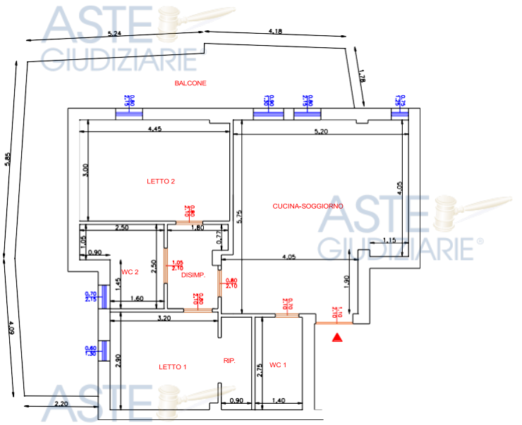
Figura 75 - Raffronto planimetrie catastali (a sinistra) e planimetrie da rilievo (a destra) – PIANO 3 – SUB 58 – BENE B
