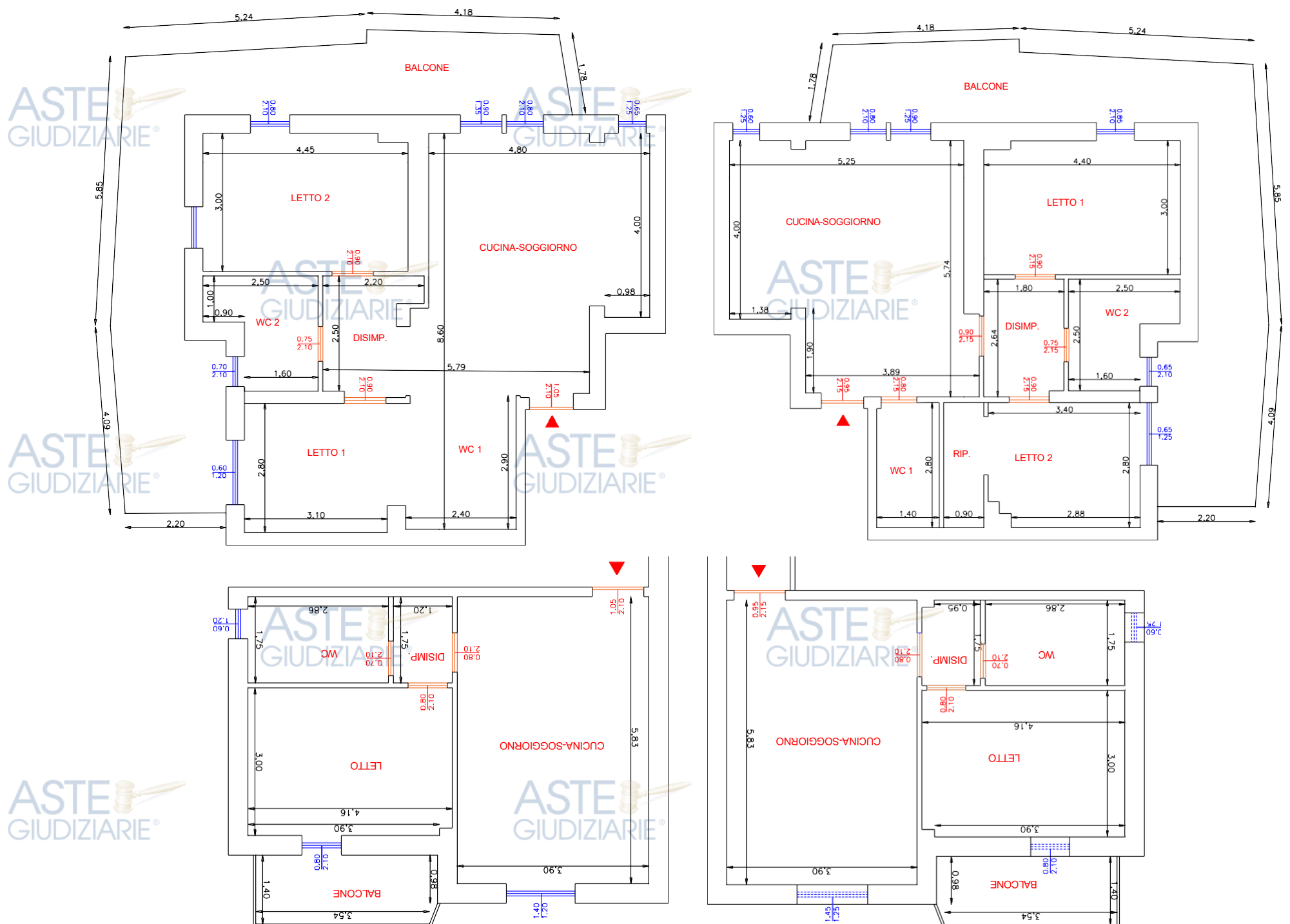
Figura 68 - Raffronto planimetrie progettuali di cui alla CLA protocollo n. 37264 del 21/04/2020 (sopra) e planimetrie d'arilevo (sotto) - PIANO SECONDO
