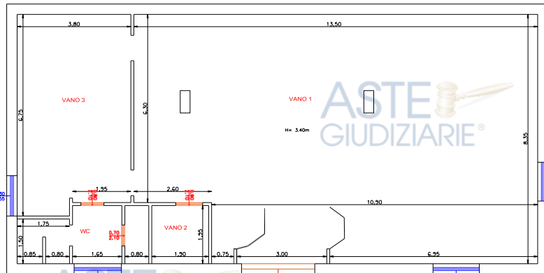
Figura 80 - Raffronto planimetrie catastali (sopra) e planimetrie da rilievo (sotto) – PART 366 - SUB 2 – BENE I
