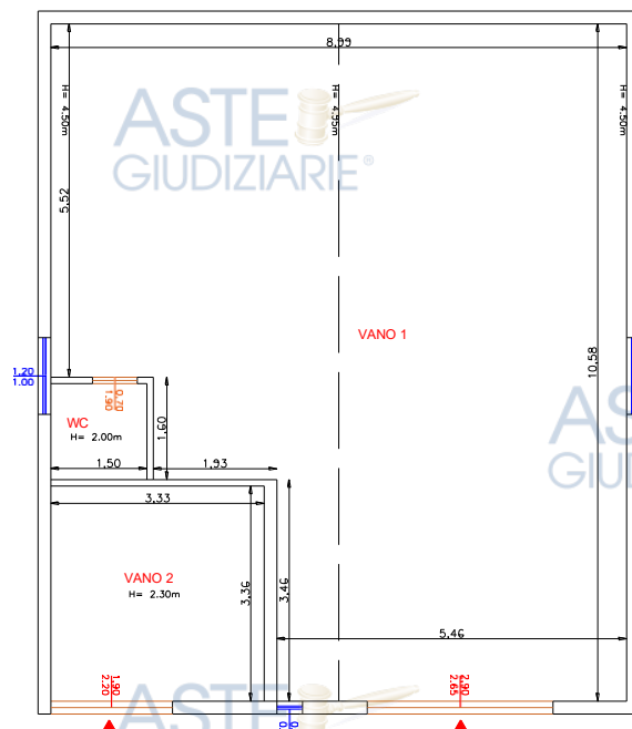
Figura 81 - Raffronto planimetrie catastali (sopra) e planimetrie da rilievo (sotto) – PART 367-368 – SUB 1101 – BENE M
