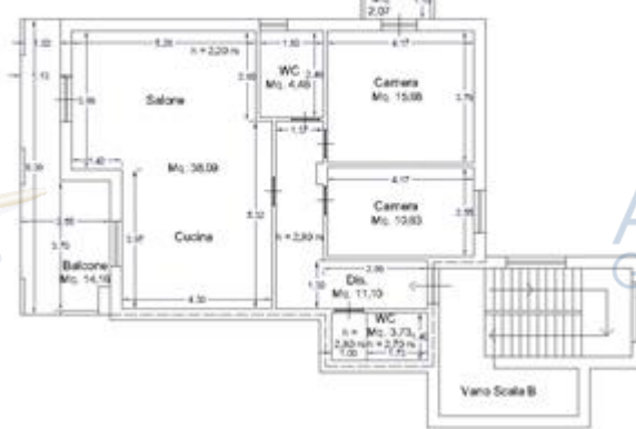
Planimetria stato di fatto
