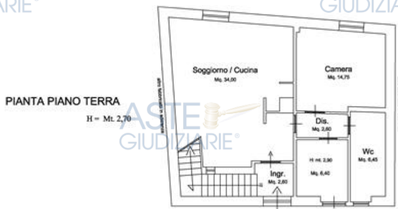
Stato di Fatto - PIANO TERRA
