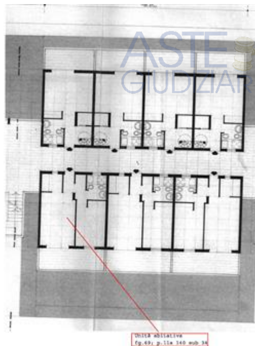
Pianta autorizzata
