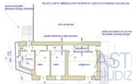
rilievo stato di fatto piano primo
