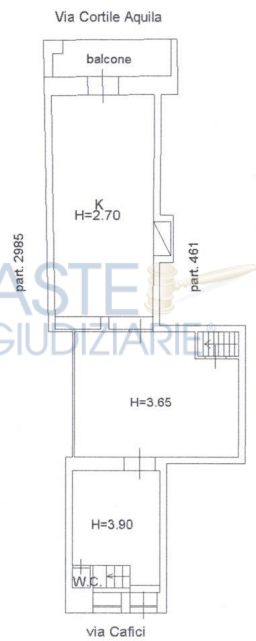
PIANO SOTTOSTRADA 2
