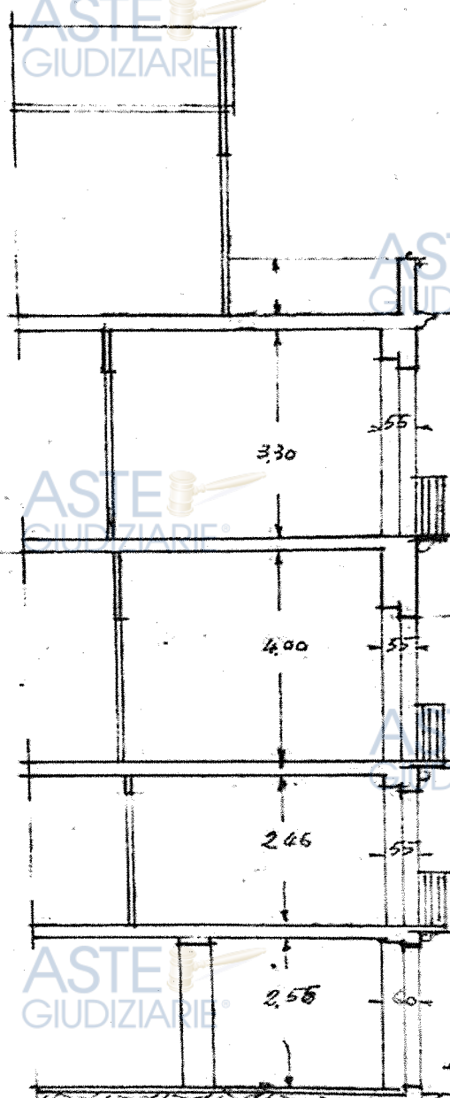
SEZIONE
