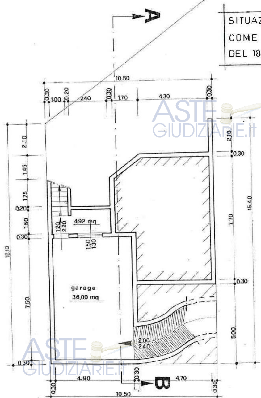
pianta seminterrato 1:100
