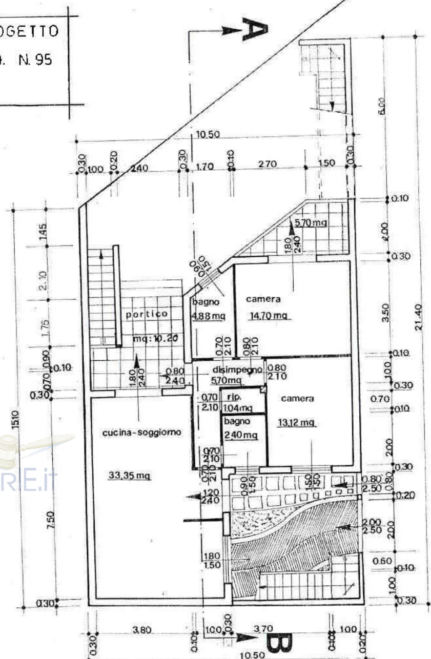
pianta piano terra 1:100
