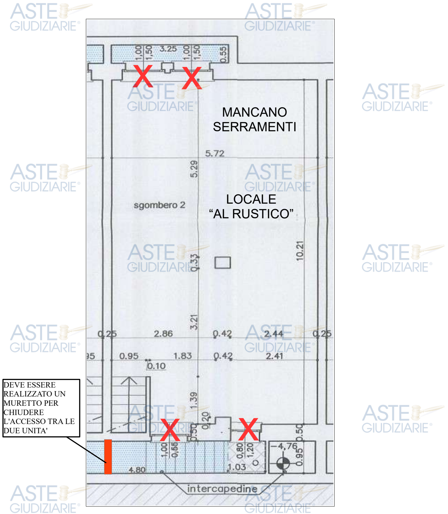
Stralcio della tavola di progetto "2V1" del P. di C. 29/2008 – piano primo interrato – locale sgombero
