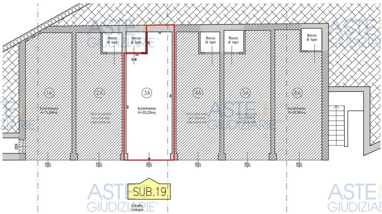
Figura 21: Estratto Tav.A03 S.C.I.A Prot. 15710 del 18.11.2025 – Piano interrato box
