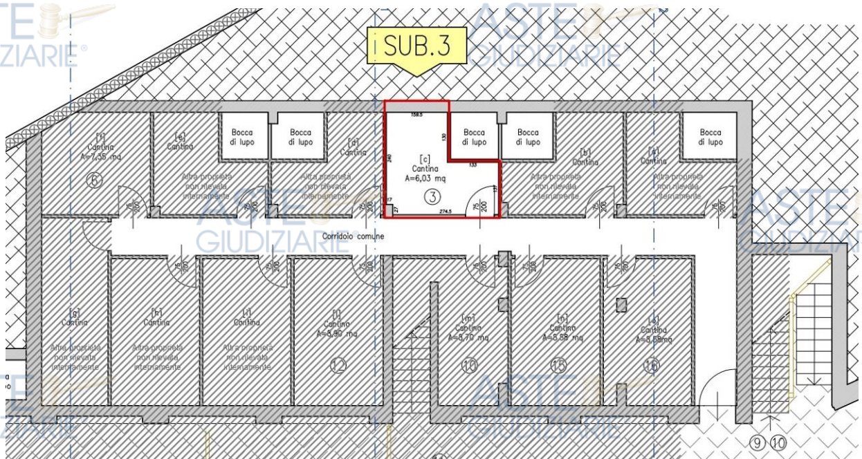
Figura 20: Estratto Tav.A03 S.C.I.A Prot. 15710 del 18.11.2025 – Piano interrato cantine
