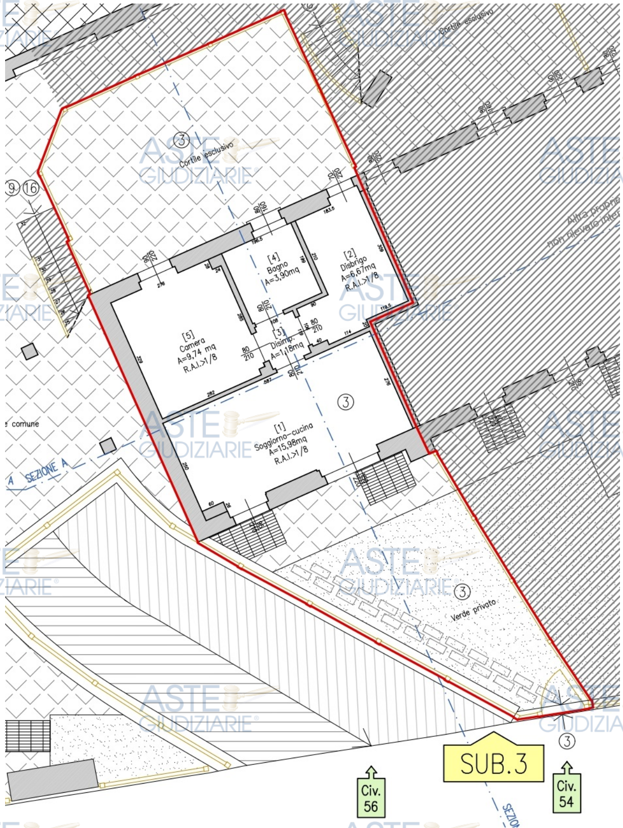
Figura 19: Estratto Tav.A03 S.C.I.A Prot. 15710 del 18.11.2025 – Piano terra
