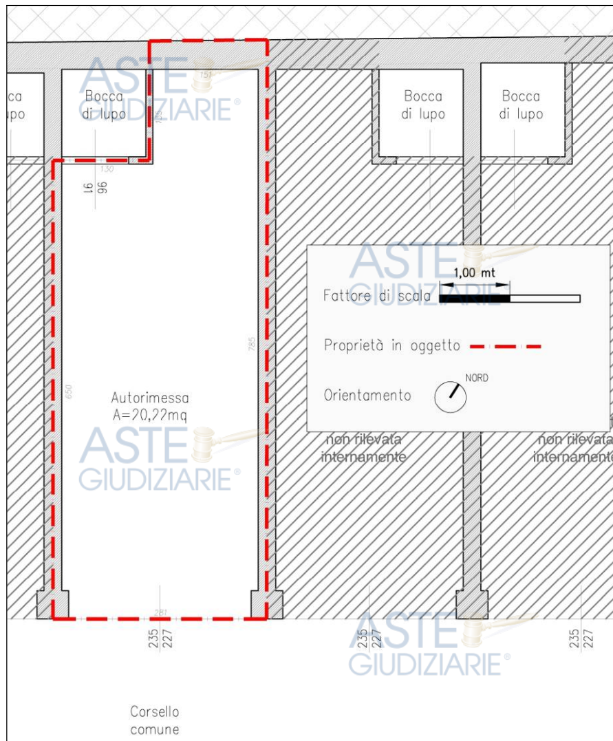
Figura 09: Piano interrato autorimesse – Pianta di rilievo autorimessa - Part. 336 sub. 19
