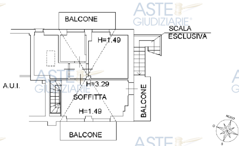
Figura 24: Part. 336 sub. 57 abitazione piano secondo
