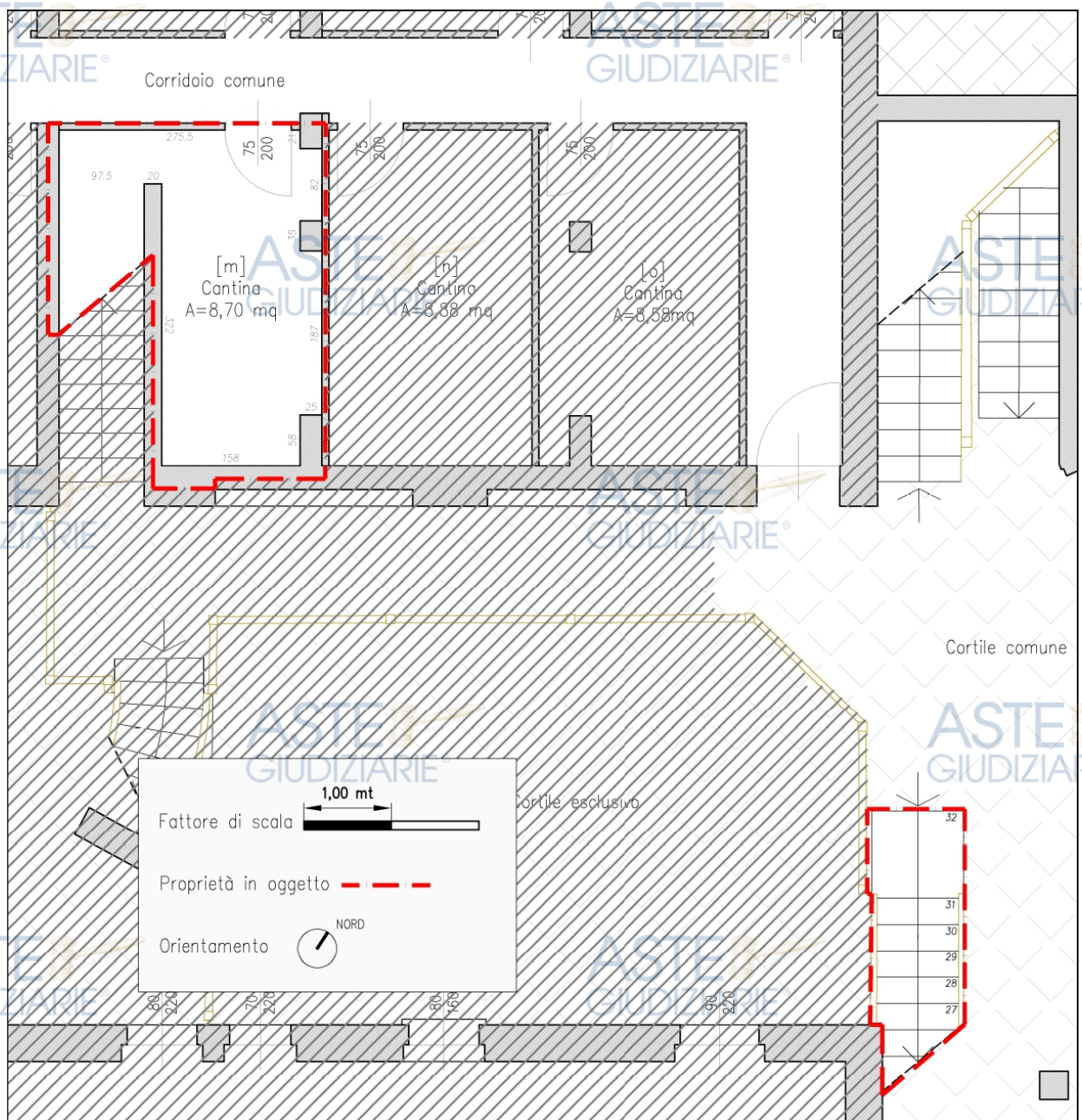
Figura 07: Piano terra/cantinato – Pianta di rilievo cantina Part. 336 sub. 58 e scala esclusiva Part. 336 sub. 57
