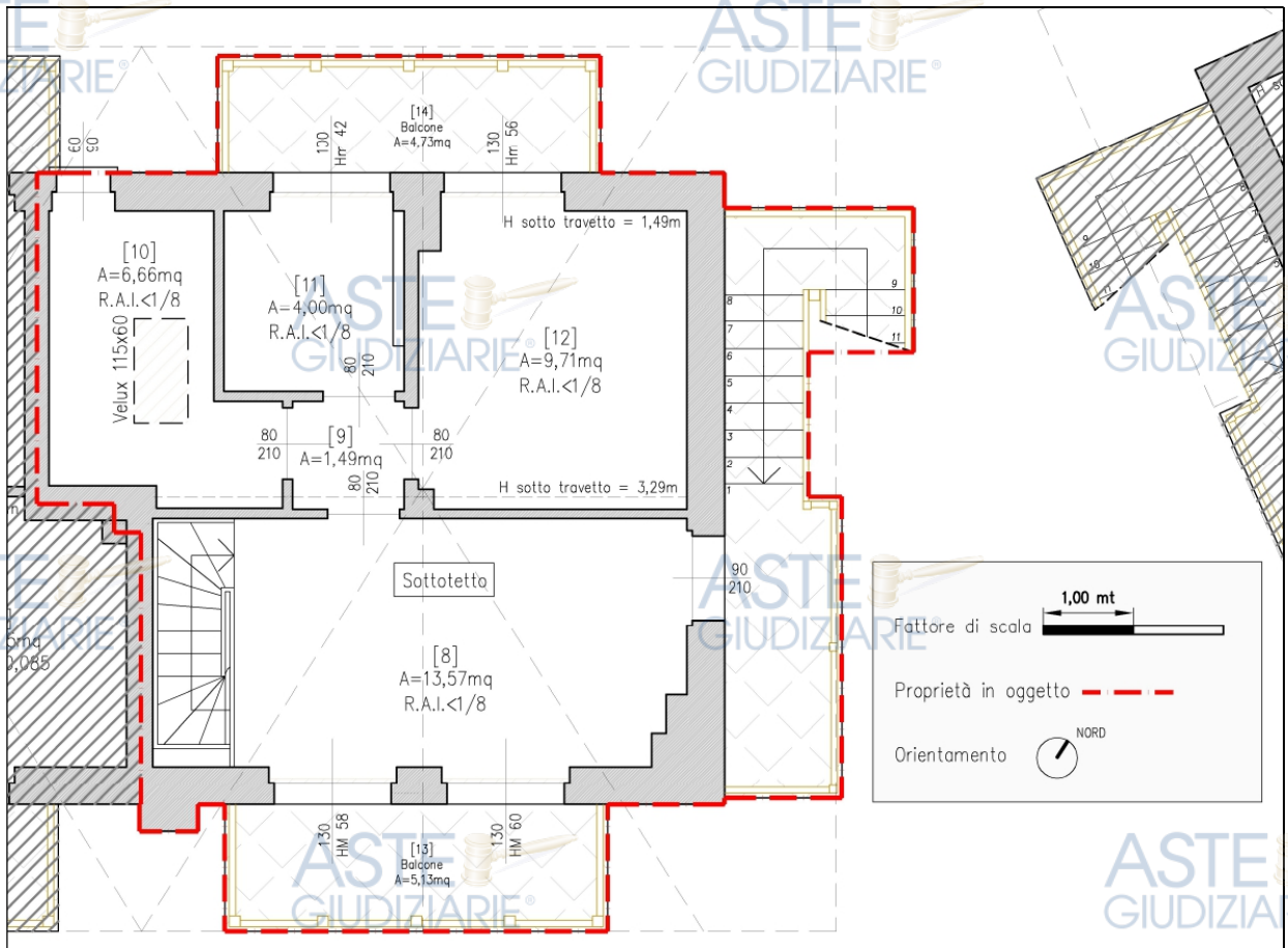
Figura 09: Piano sottotetto – Pianta di rilievo abitazione - Part. 336 sub. 57
