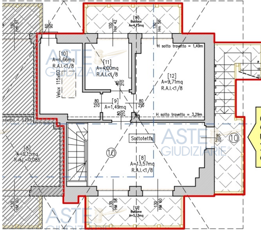
Figura 29: Estratto Tav.A04 S.C.I.A Prot. 15712 del 18.11.2025 – Piano sottotetto
