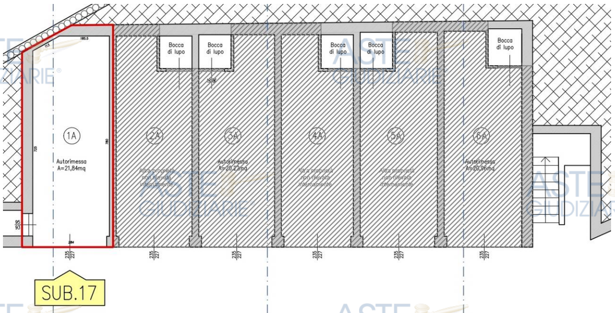
Figura 30: Estratto Tav.A03 S.C.I.A Prot. 15712 del 18.11.2025 – Piano interrato box
