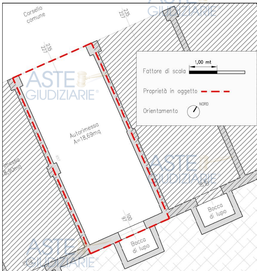
Figura 11: Piano interrato autorimesse – Pianta di rilievo autorimessa - Part. 336 sub. 30
