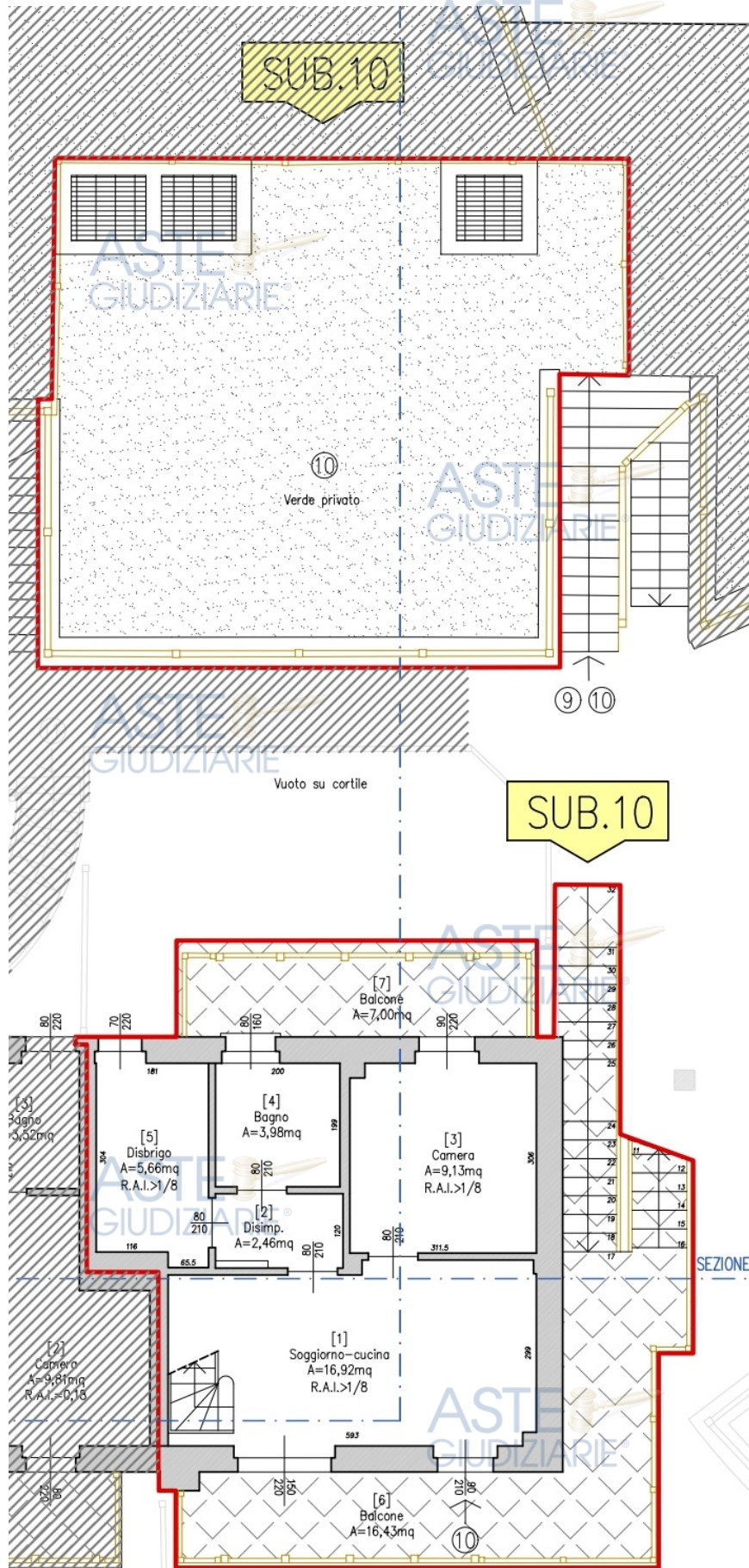
Figura 28: Estratto Tav.A04 S.C.I.A Prot. 15712 del 18.11.2025 – Piano primo
