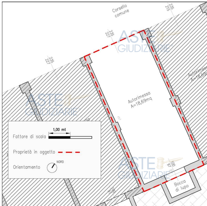
Figura 10: Piano interrato autorimesse – Pianta di rilievo autorimessa - Part. 336 sub. 29
