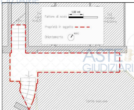
Figura 07: Piano terra/cantinato – Pianta di rilievo corte esclusiva/scala - Part. 336 sub. 11
