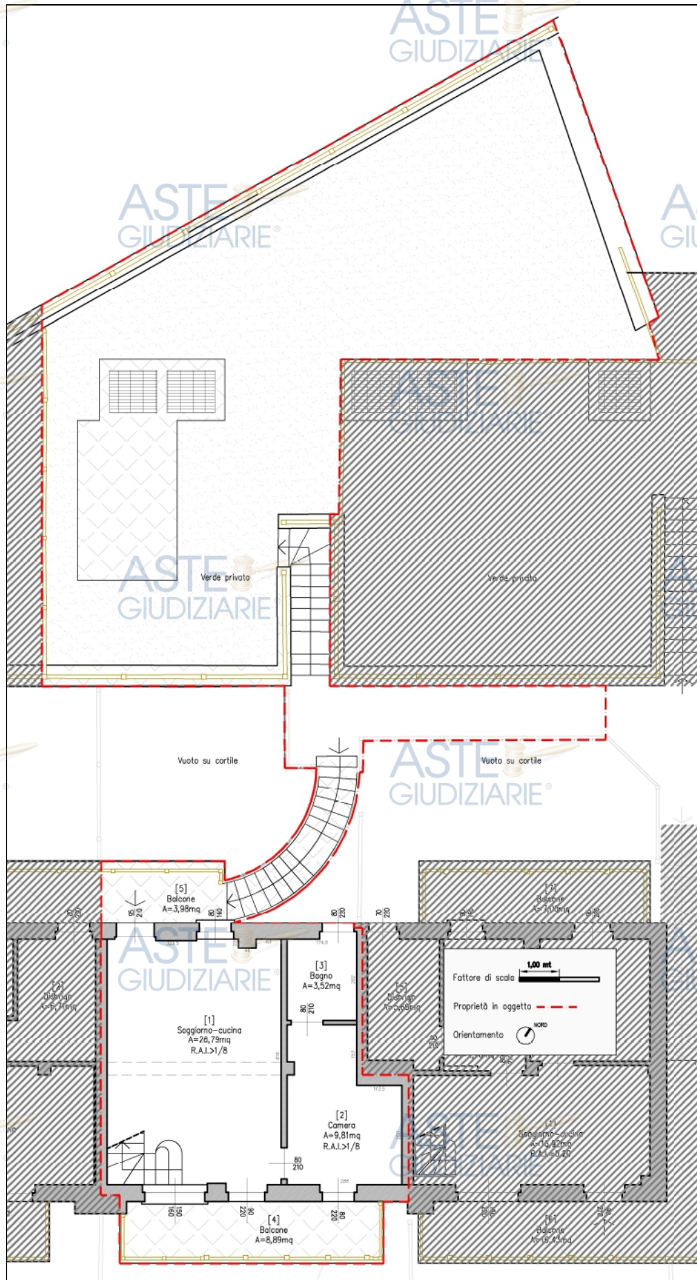
Figura 08: Piano primo – Pianta di rilievo abitazione e giardino - Part. 336 sub. 11
