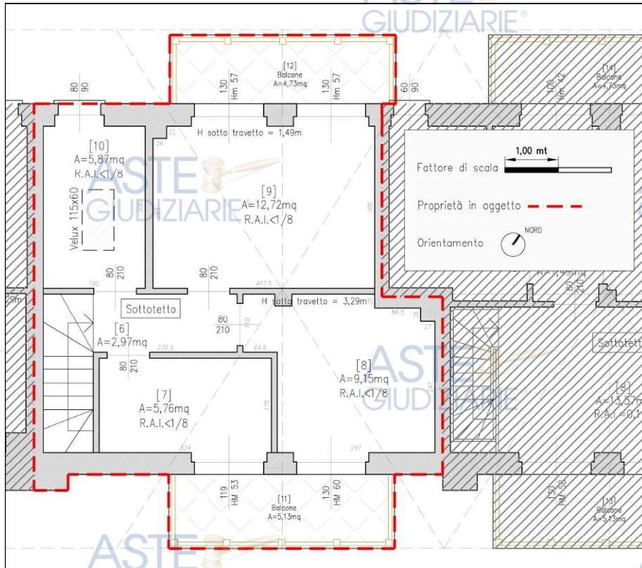
Figura 09: Piano sottotetto – Pianta di rilievo abitazione - Part. 336 sub. 11
