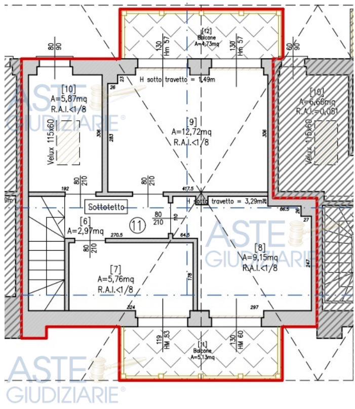
Figura 27: Estratto Tav.A04 S.C.I.A Prot. 15713 del 18.11.2025 – Piano sottotetto
