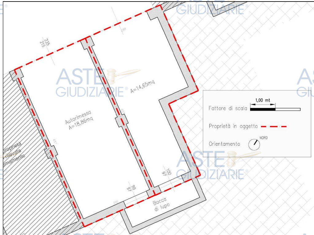
Figura 11: Piano interrato autorimesse – Pianta di rilievo autorimesse - Part. 336 sub. 59-26
