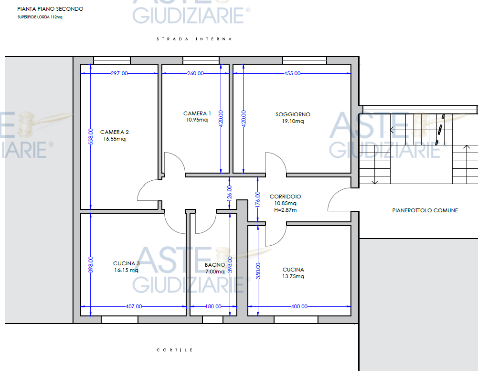
Planimetria quotata di rilievo dell'unità immobiliare al piano secondo
