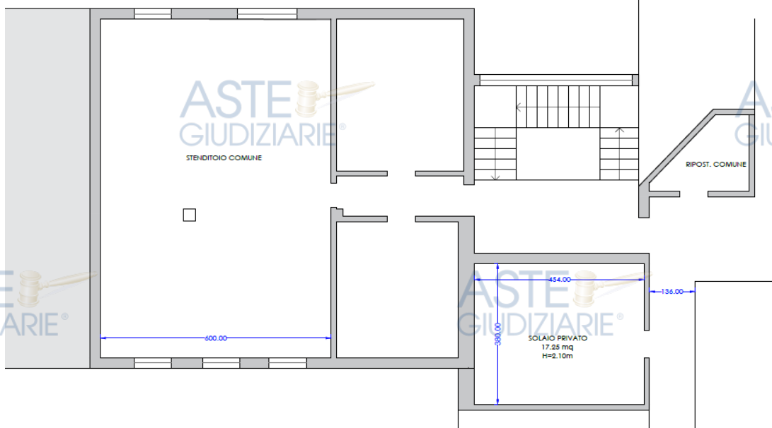
Planimetria quotata di rilievo del piano sottotetto
